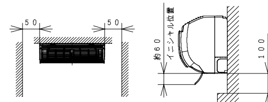
室内機サービススペース
