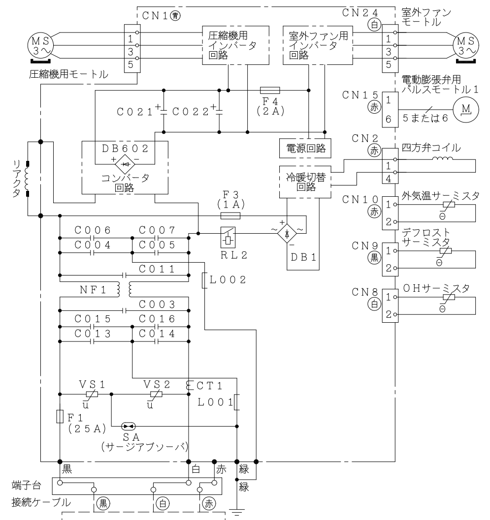
配線図 RAC-E40J2
