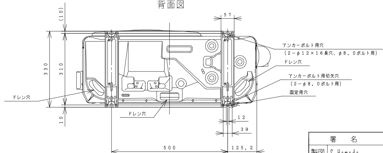
背面図
