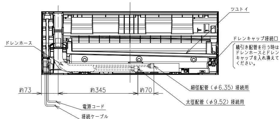
背面図
