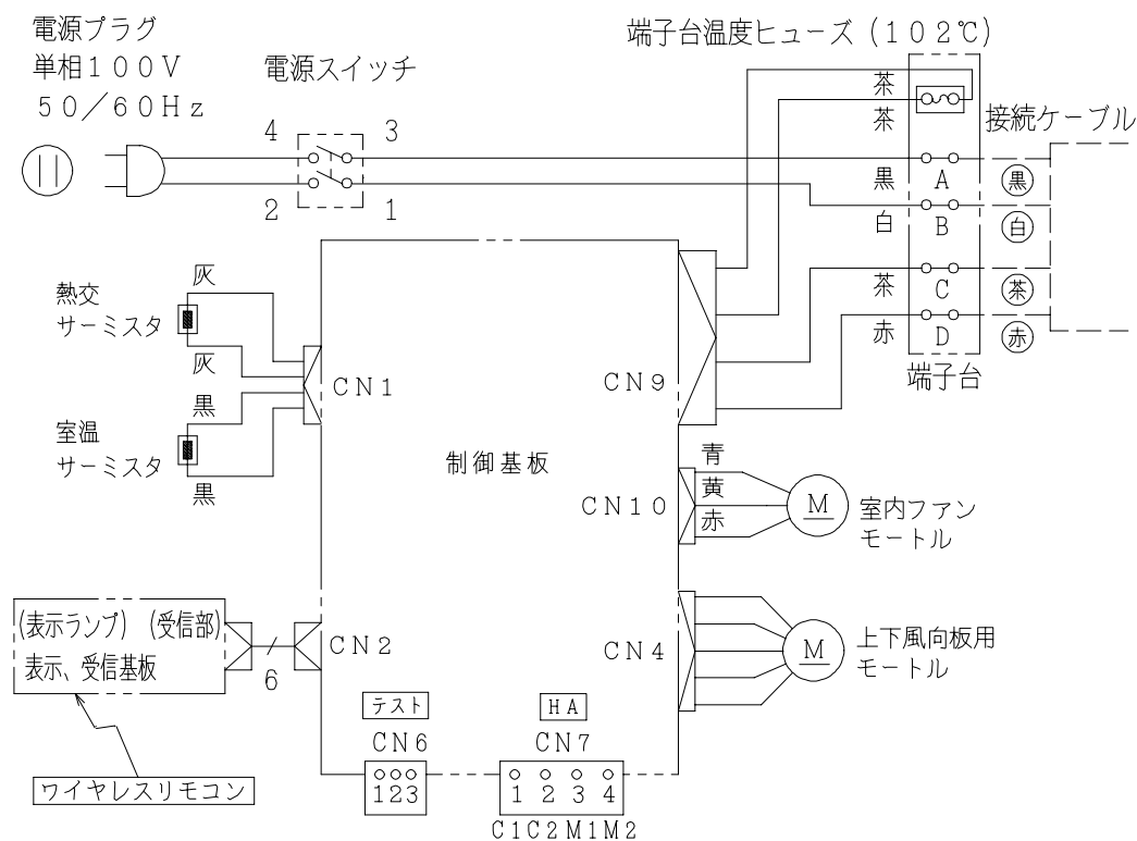
配線図 RAS-C25KX
