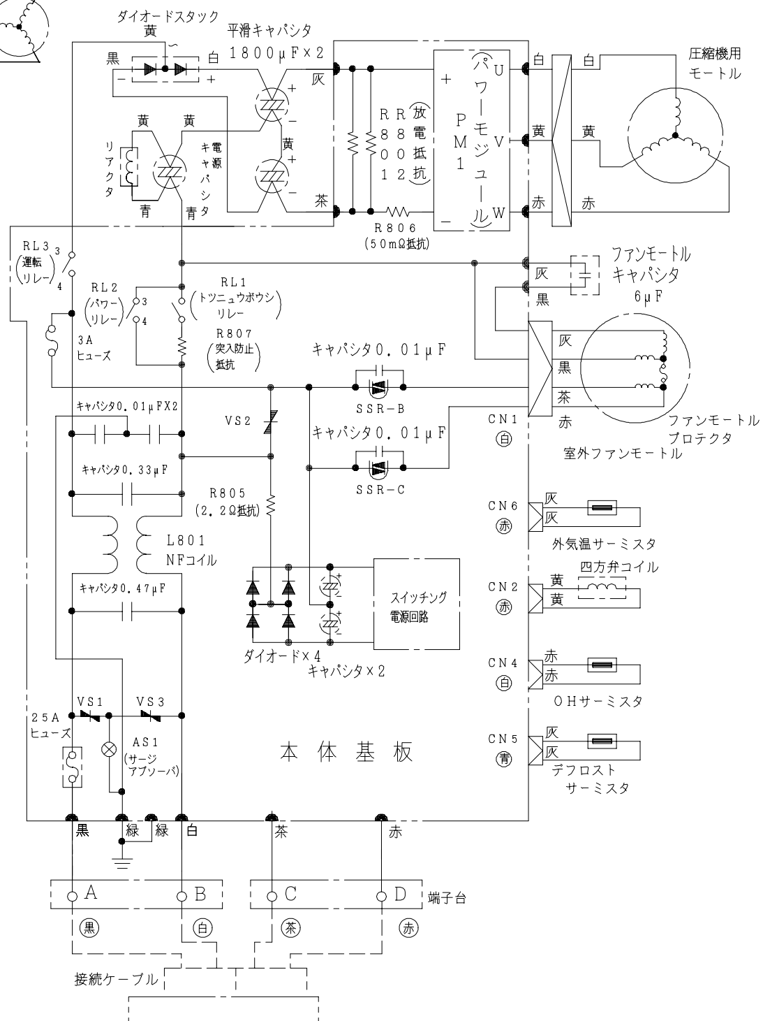
配線図 RAC-258KX
