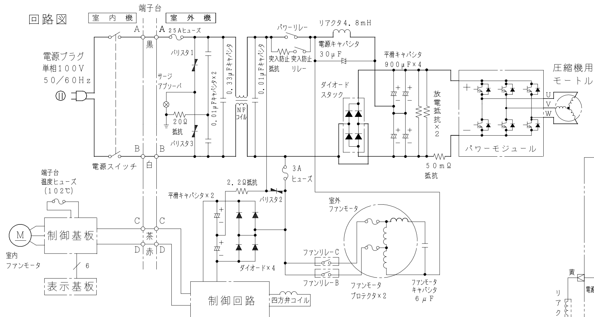
配線図 RAS-C25JX
