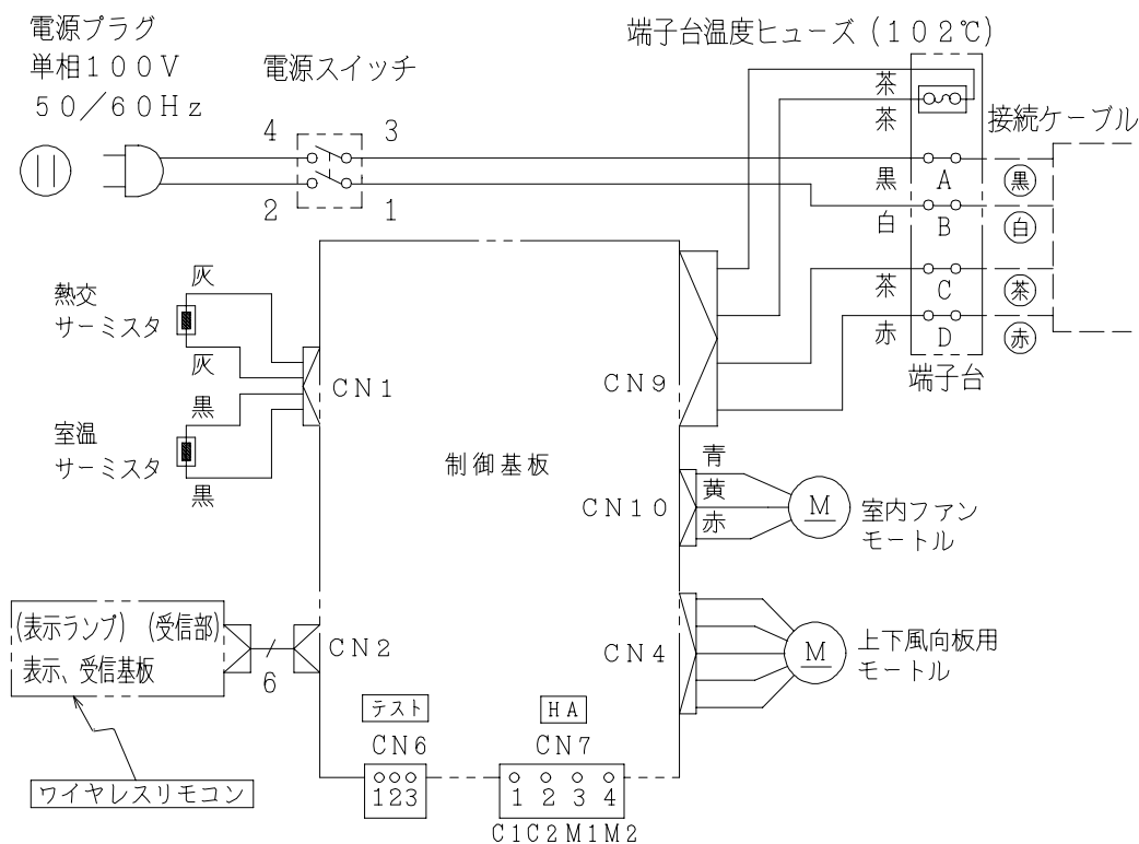
配線図 RAS-C25JX
