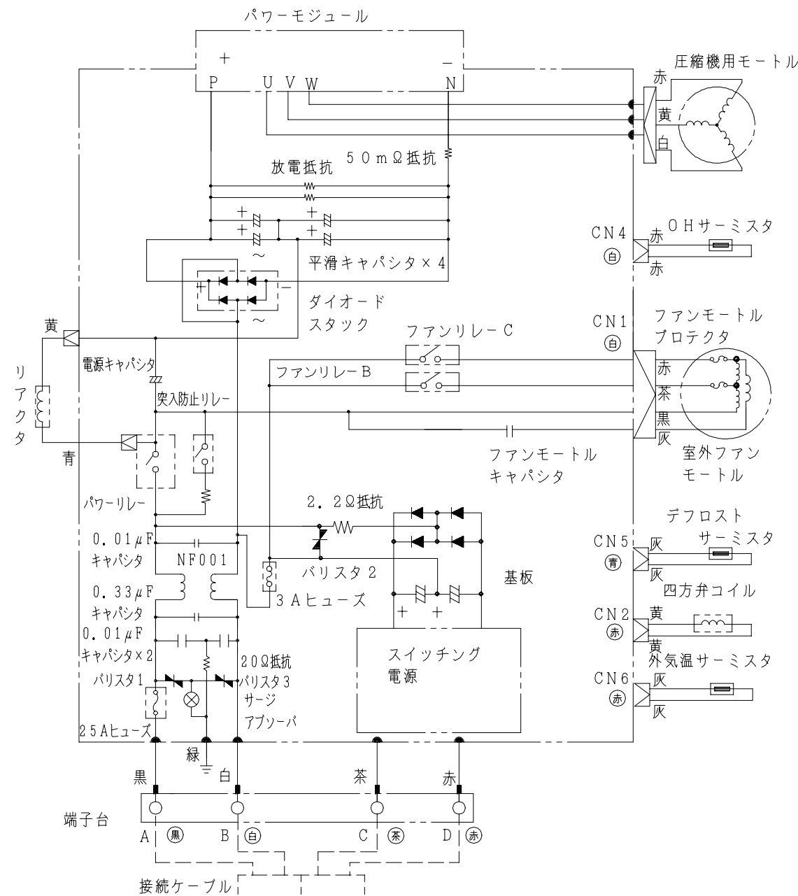
配線図 RAC-258JX
