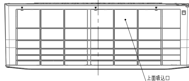
日立ルームエアコン 壁掛BZシリーズ 室内ユニット 寸法図
