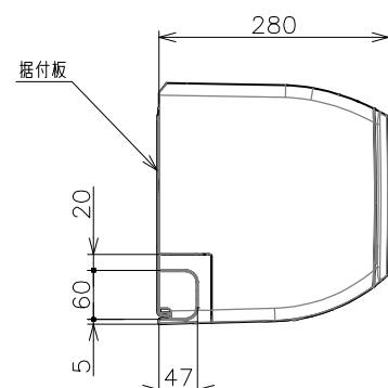
日立ルームエアコン 壁掛BZシリーズ 室内ユニット 寸法図
