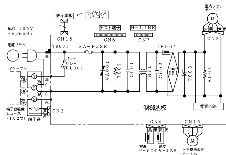
配線図 R A S - A C 2 5 Z
