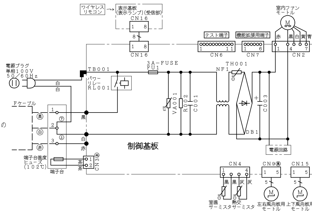
配線図 R A S - A C 2 5 G
