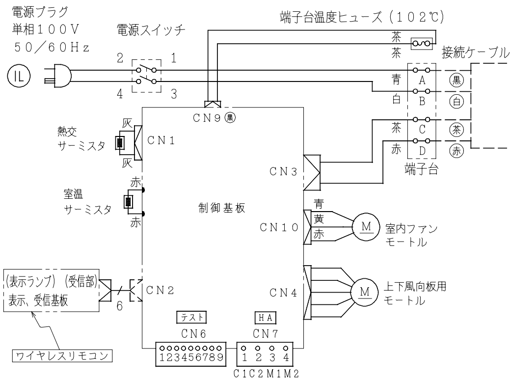
配線図 RAS-A28GX
