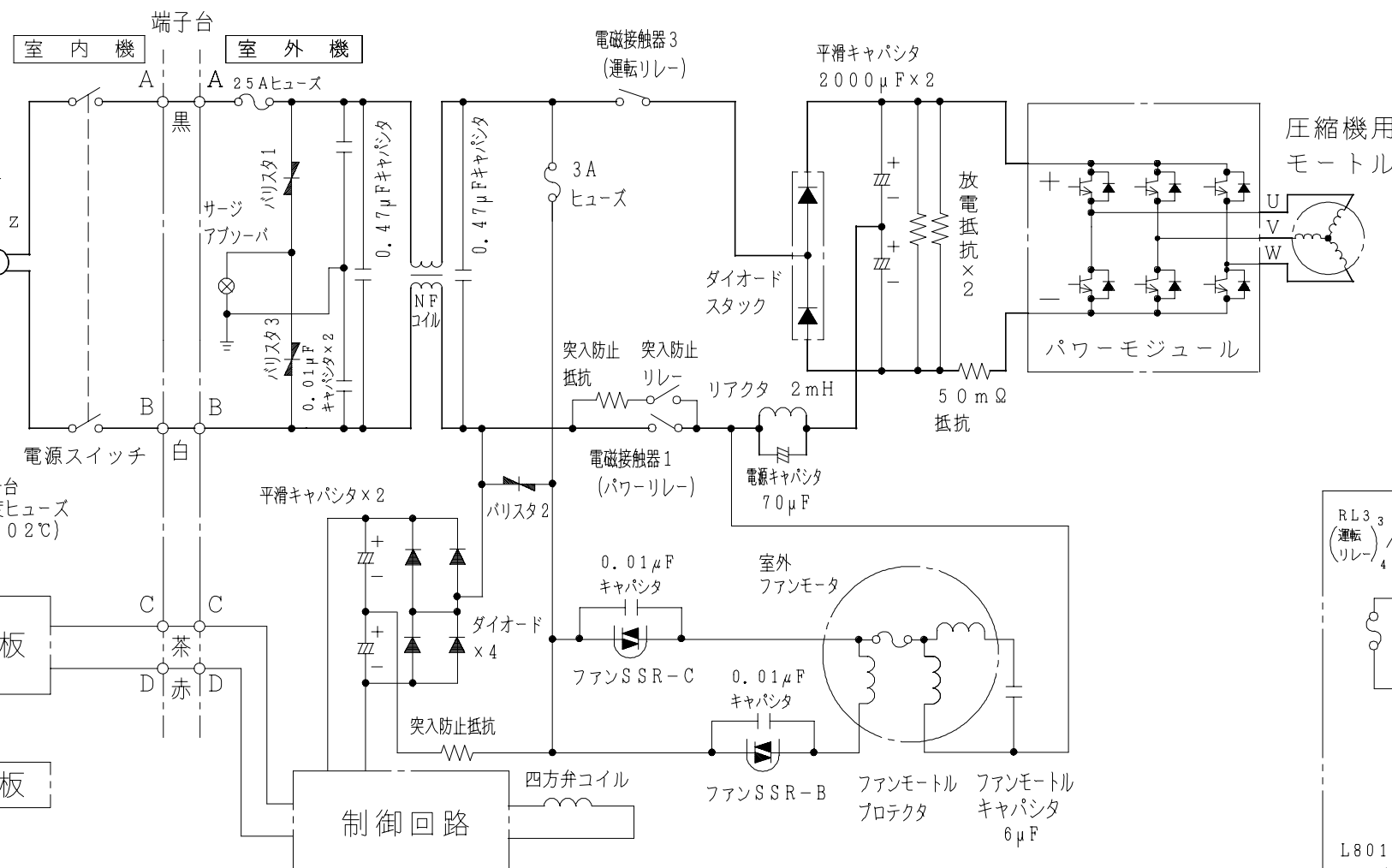
配線図 RAS-A28GX
