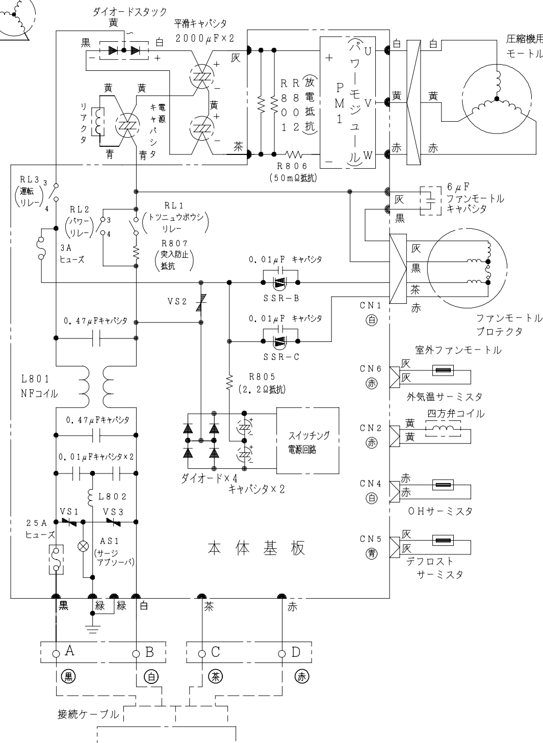
配線図 RAC-287GX
