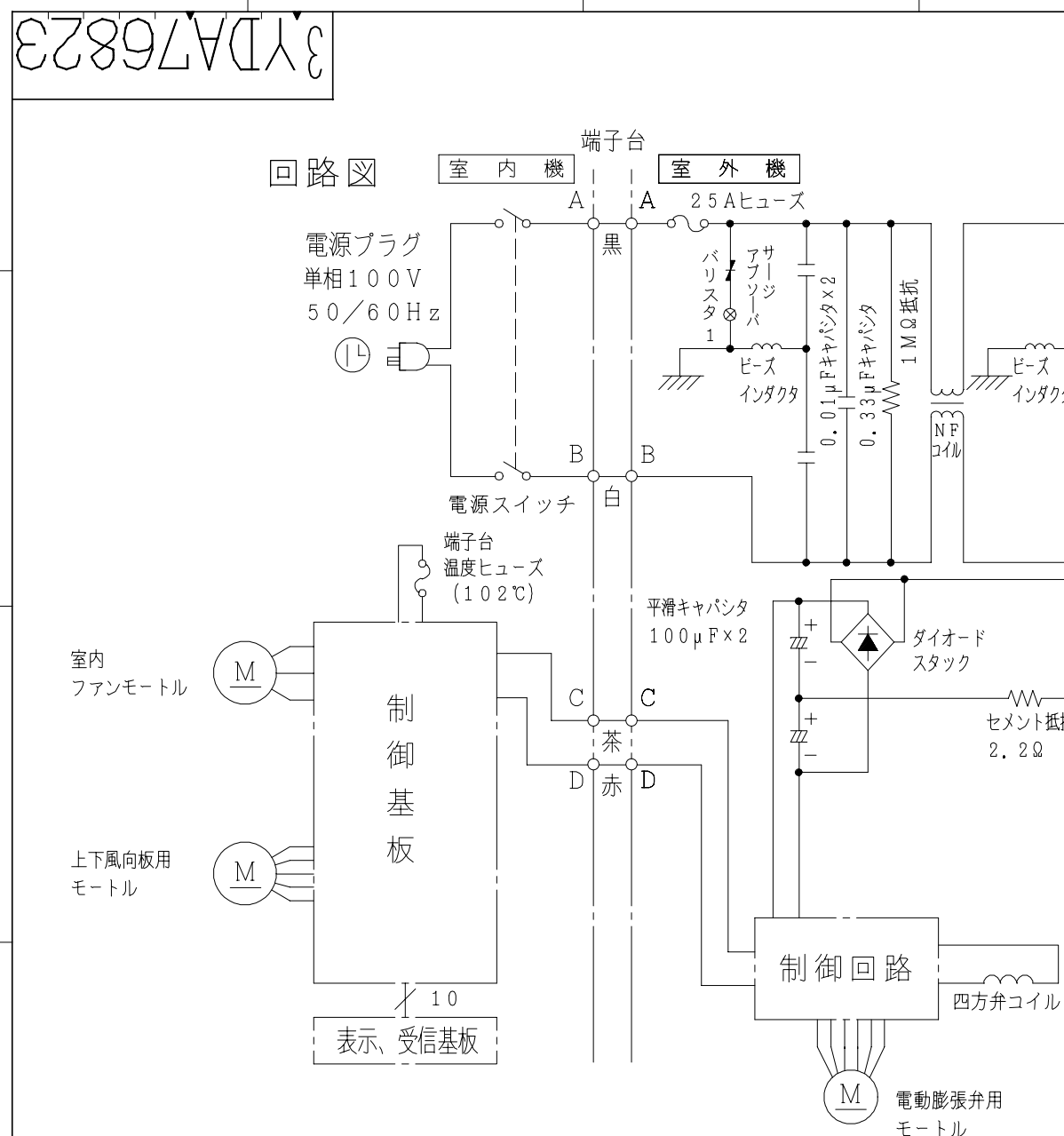
配線図 RAS-32SKX
