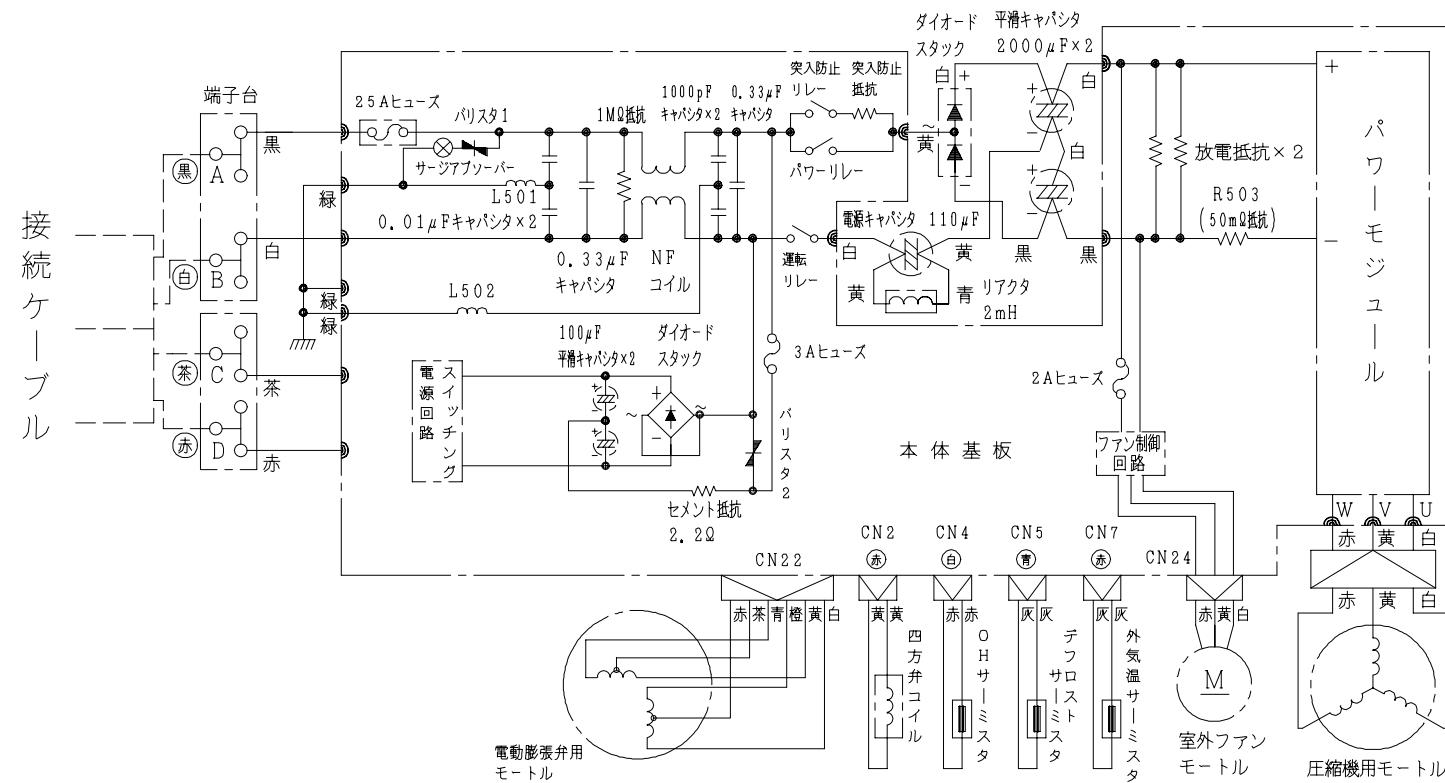
配線図 RAC-32HKX
