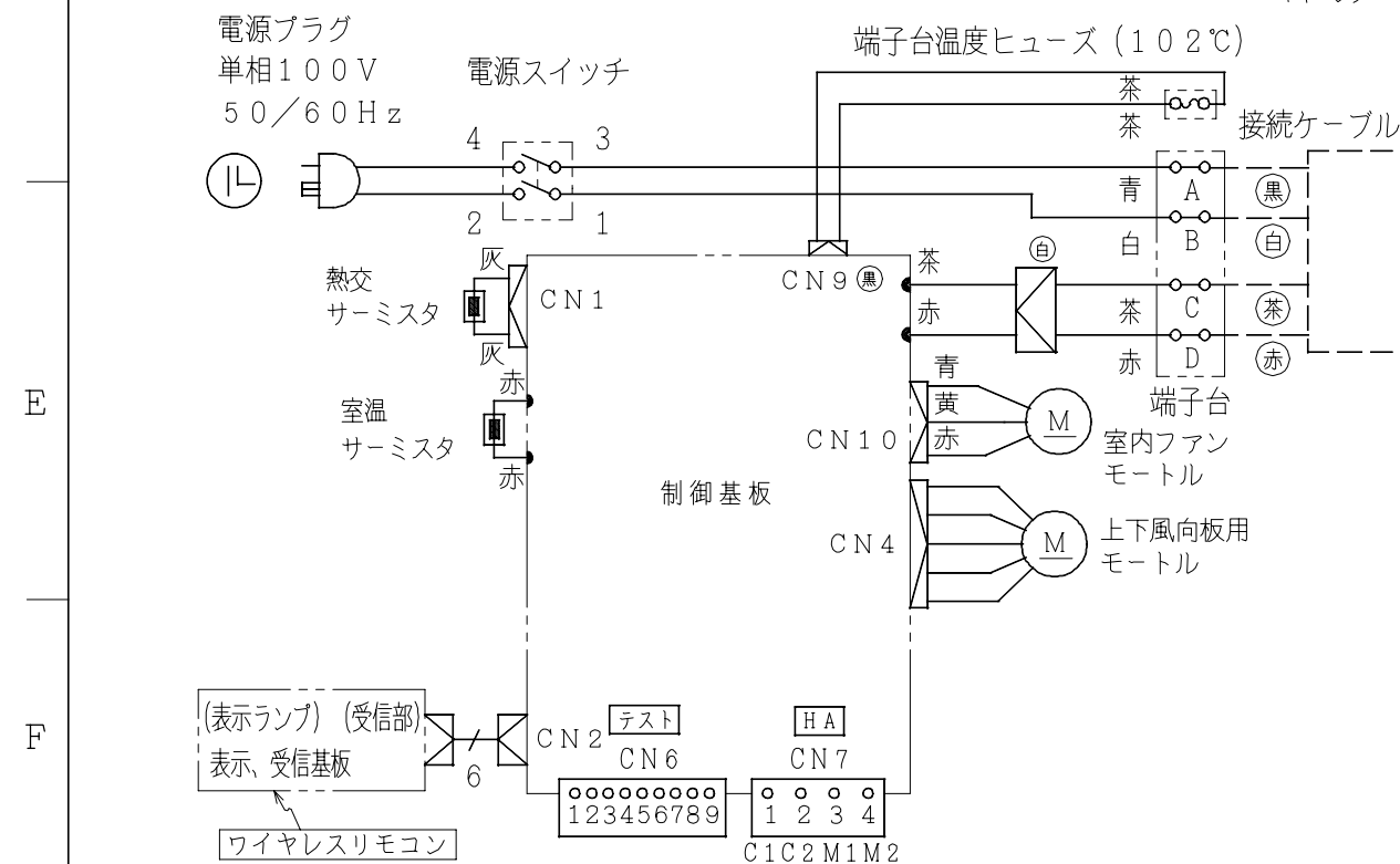
配線図 RAS-32HGX
