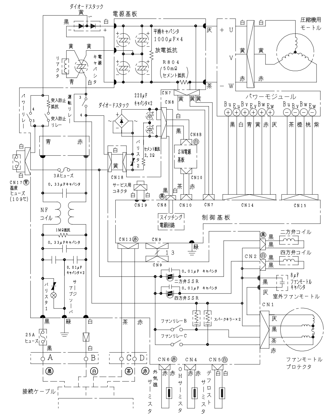
配線図 R A C - 3 2 H S G X
