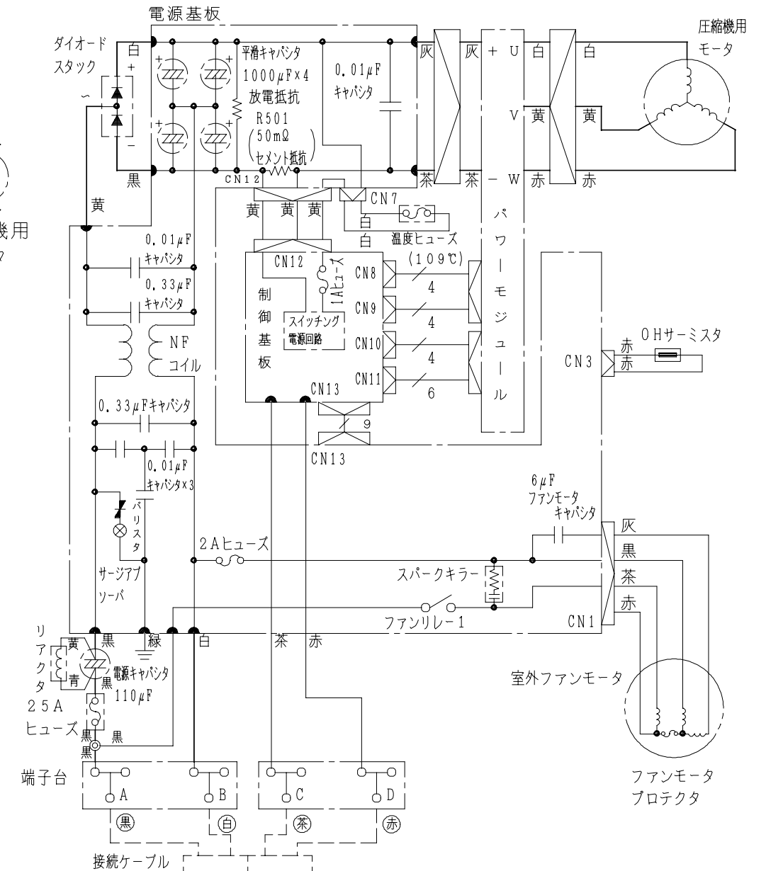
配線図 R A C - 3 2 E E M
