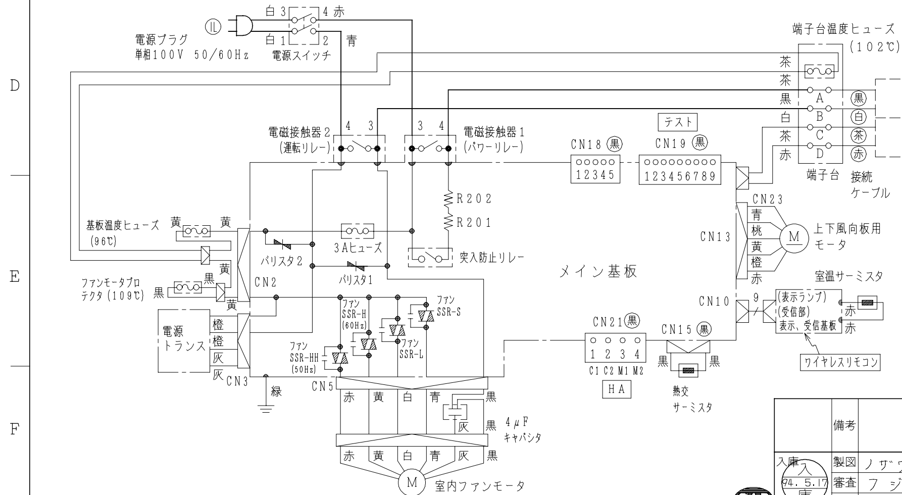
配線図 RAS-32EEM
