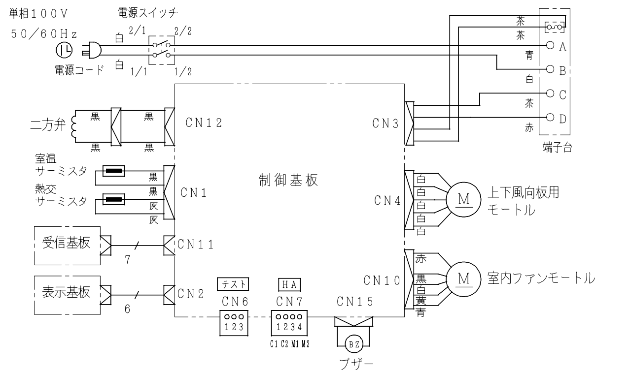
配線図 RAS-329LX
