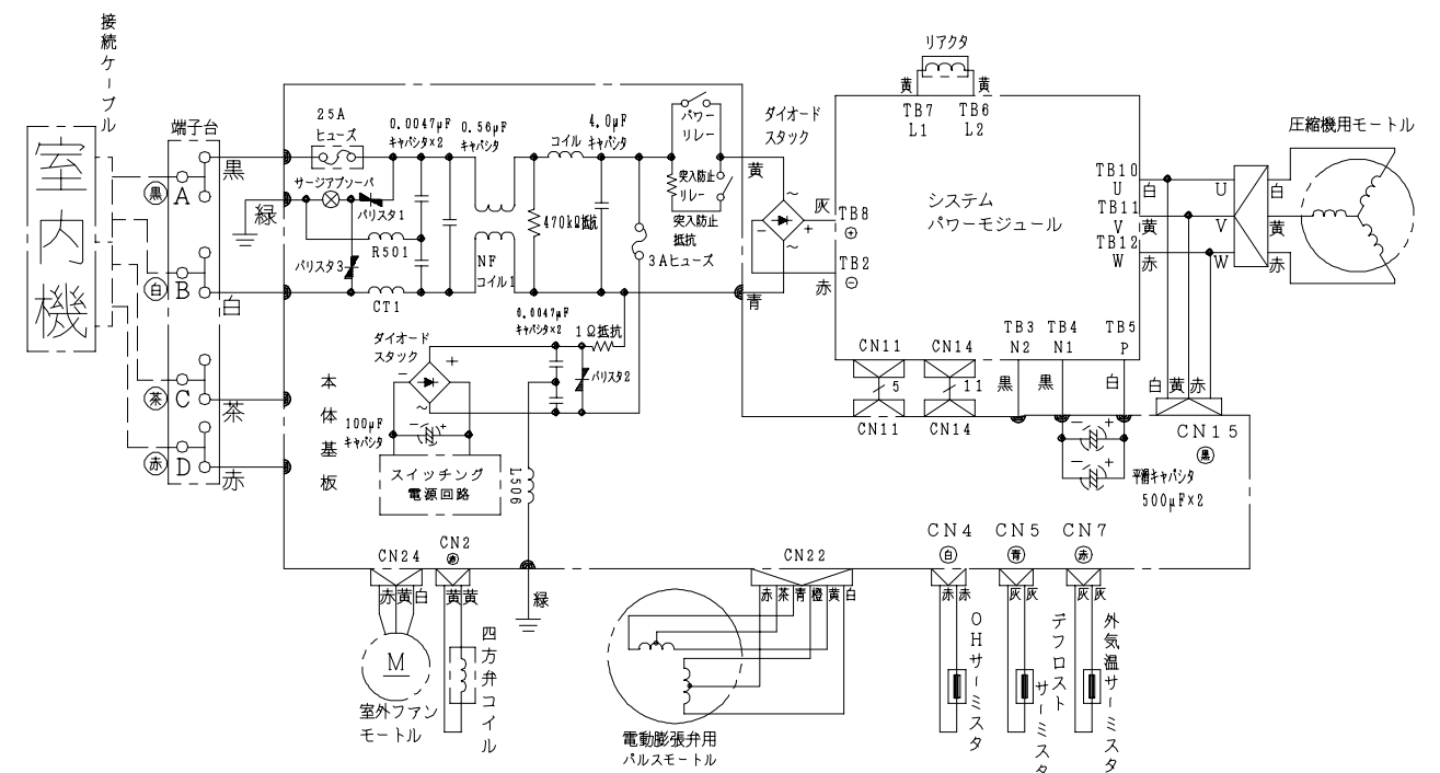
配線図 R A C - 3 2 9 L X
