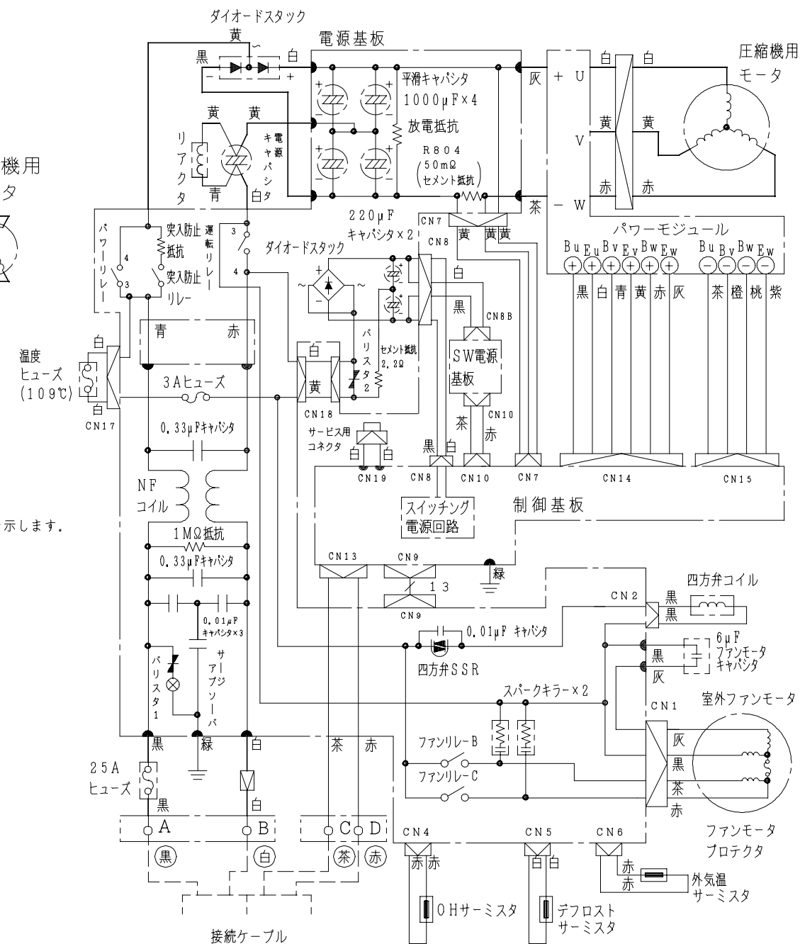
配線図 RAC-28HSFX
