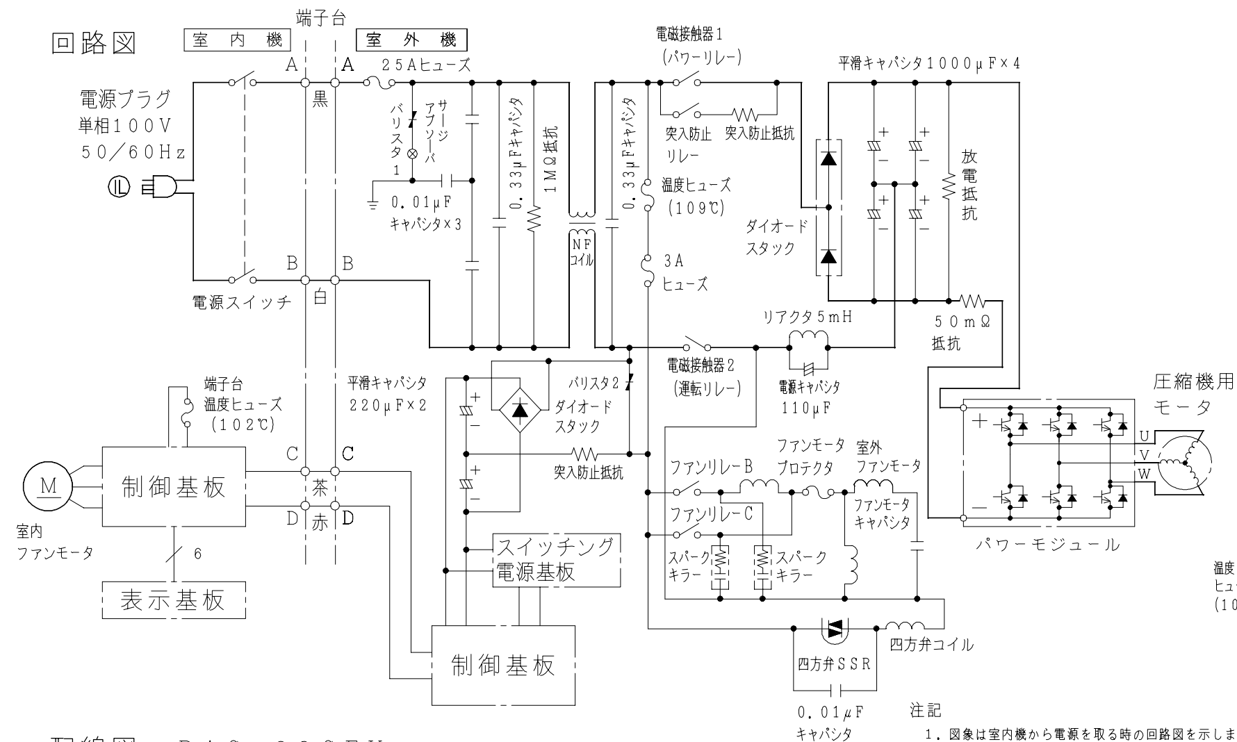
配線図 RAS-28SFX
