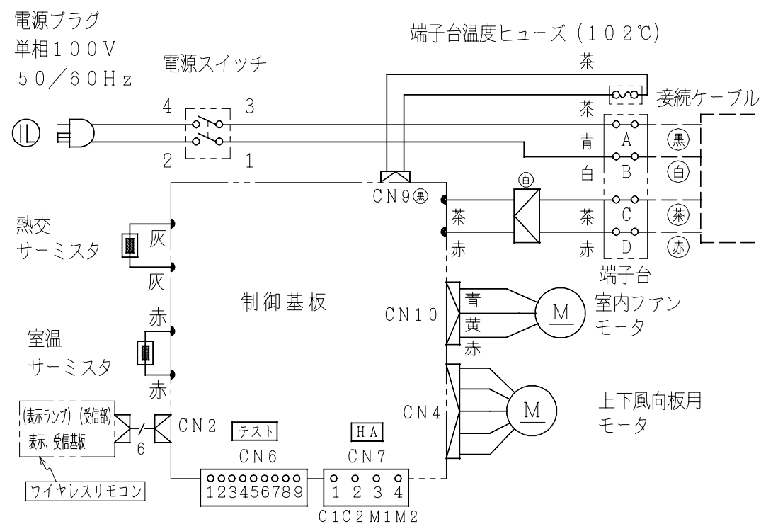
配線図 RAS-28SFX
