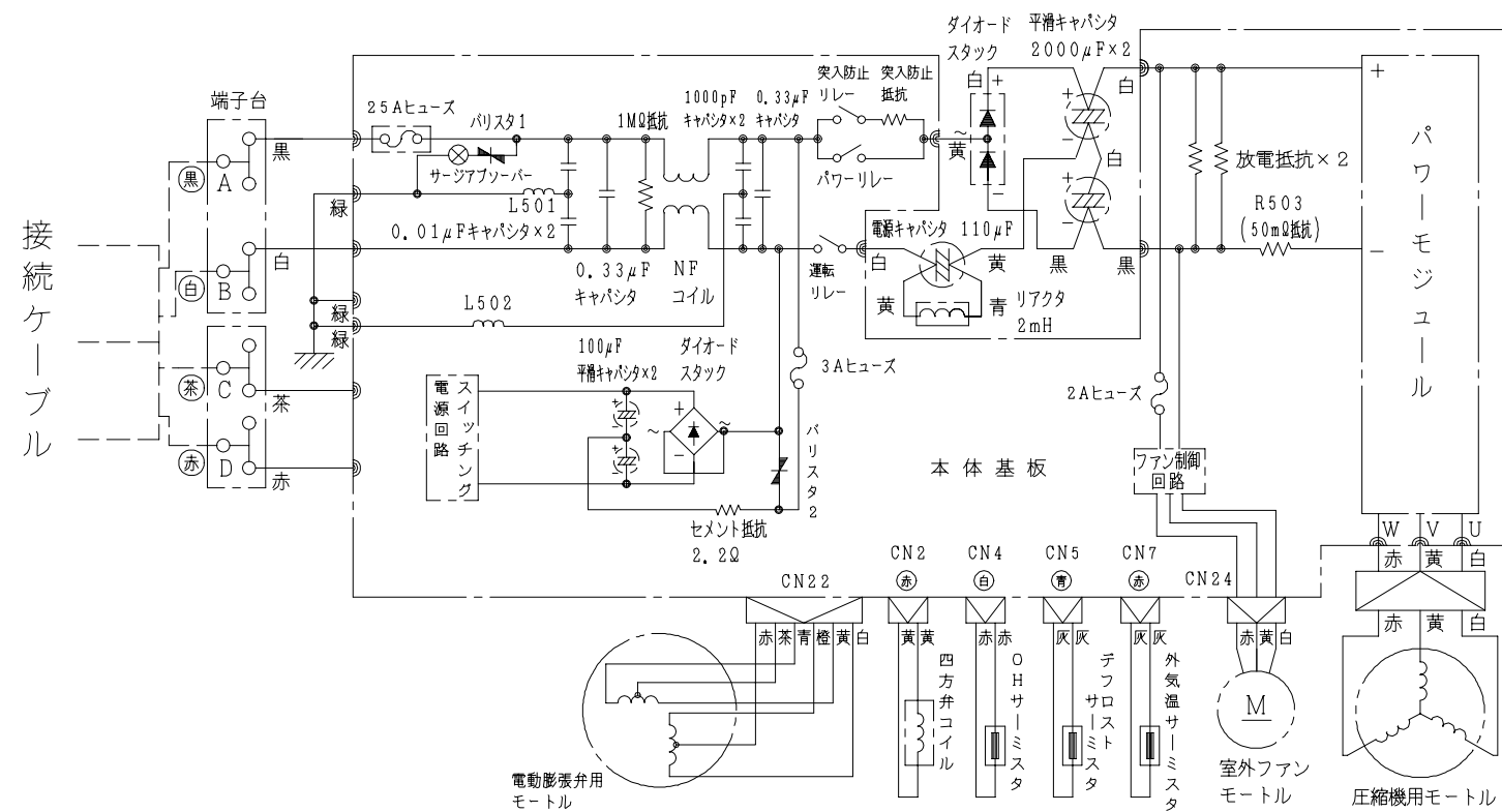
配線図 RAC-28KXM
