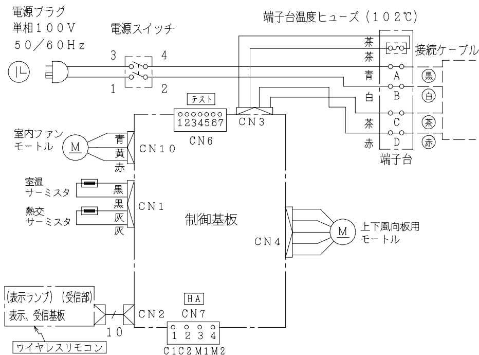
配線図 RAS-28KXM
