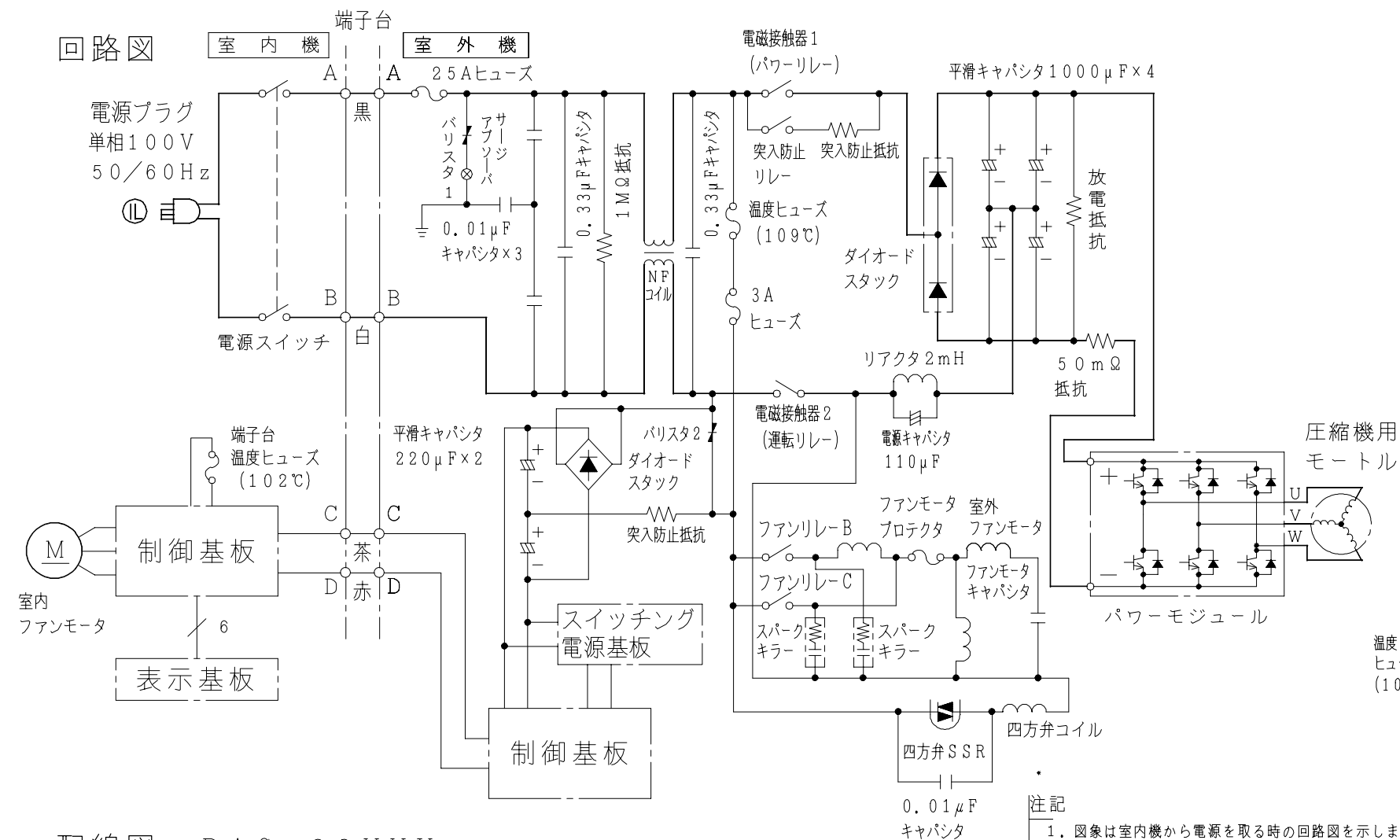
配線図 RAS-28HHX
