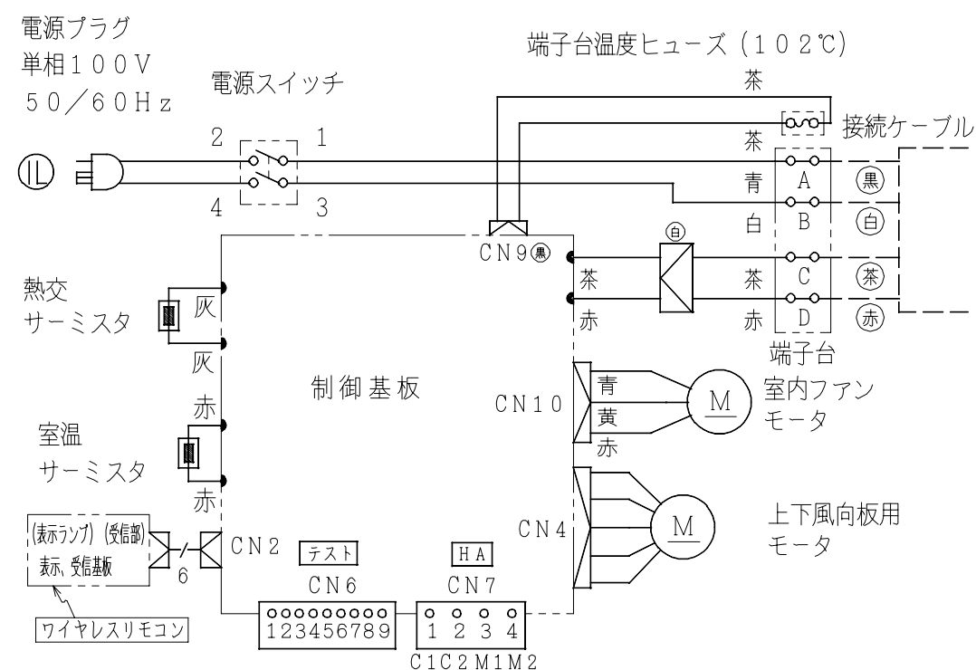
配線図 RAS-28HHX
