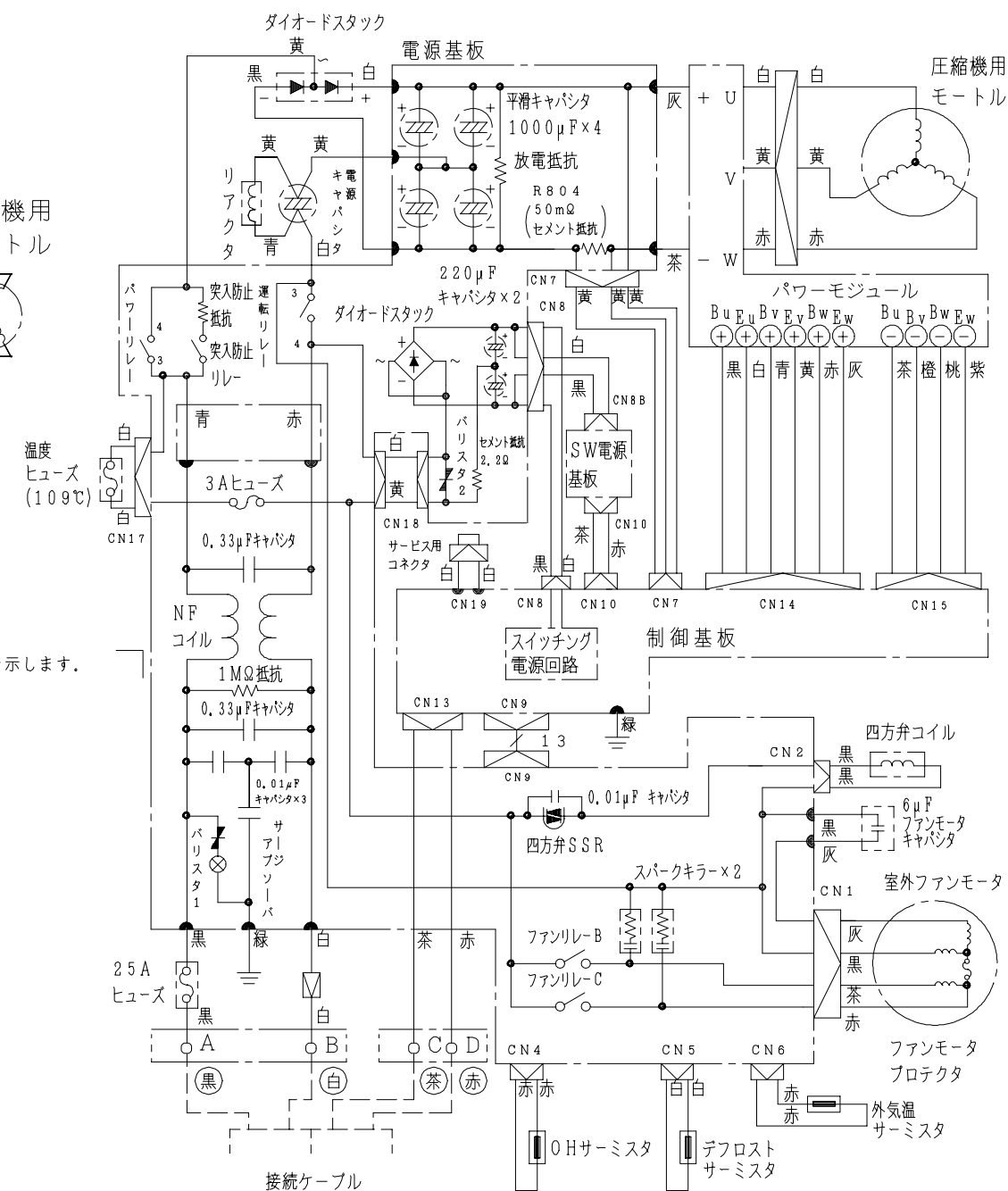
配線図 R A C - 2 8 H H X
