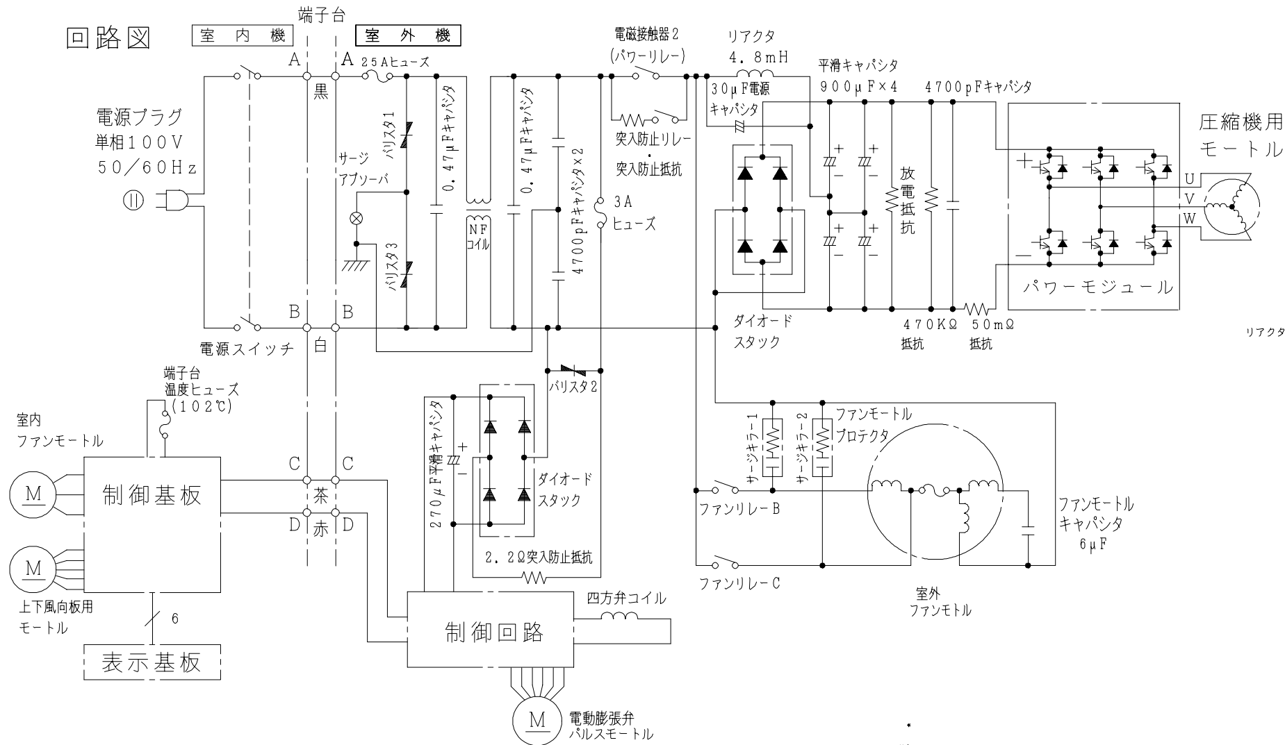
配線図 RAS-28FNX
