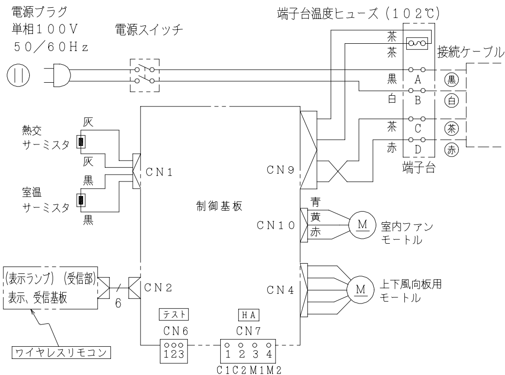
配線図 RAS-28FNX
