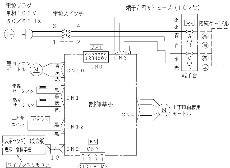
配線図 RAS-289JX
