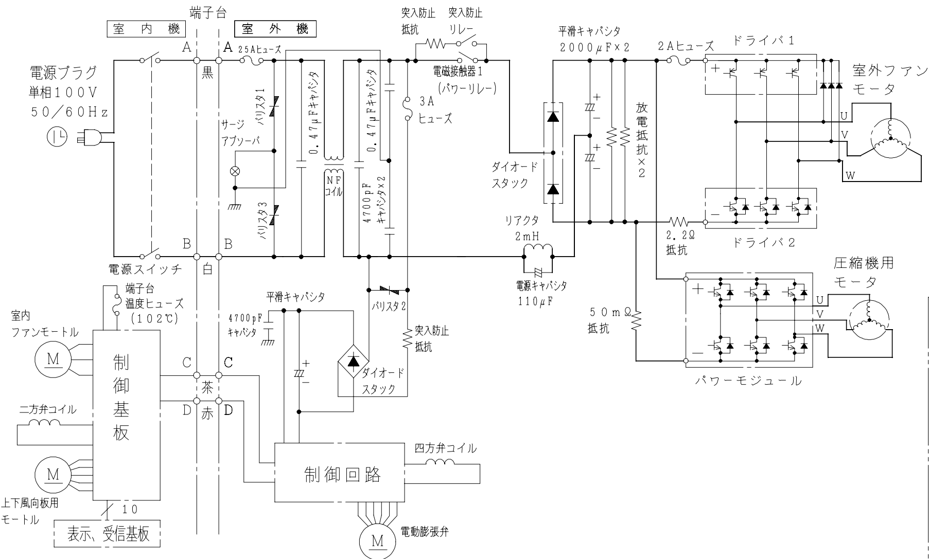
回路図
