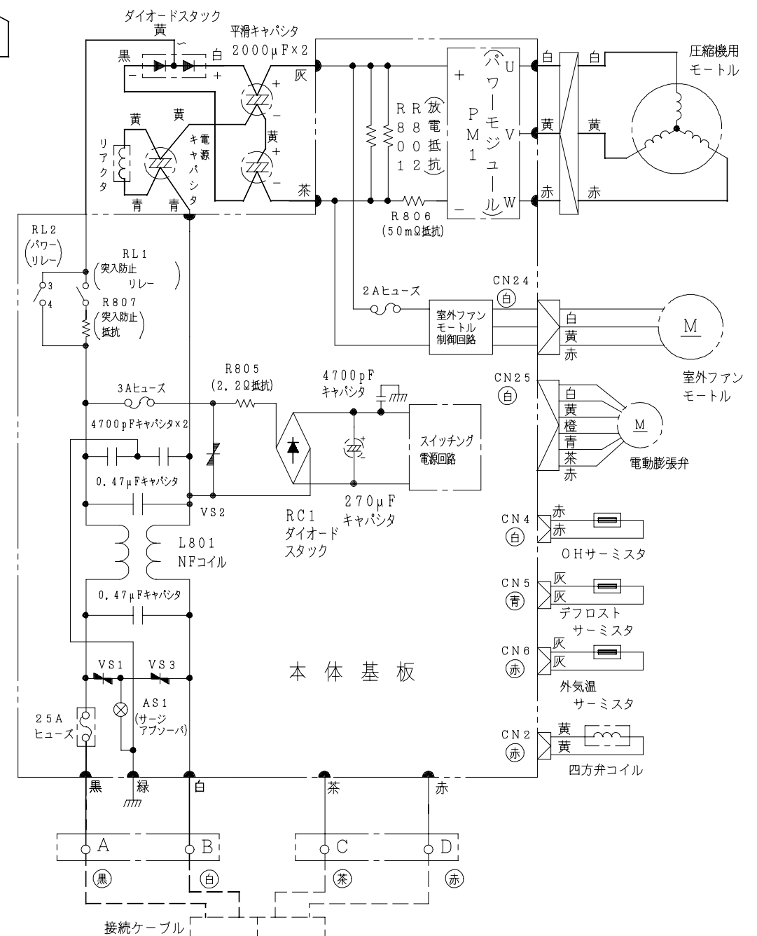
配線図 RAC-289JX
