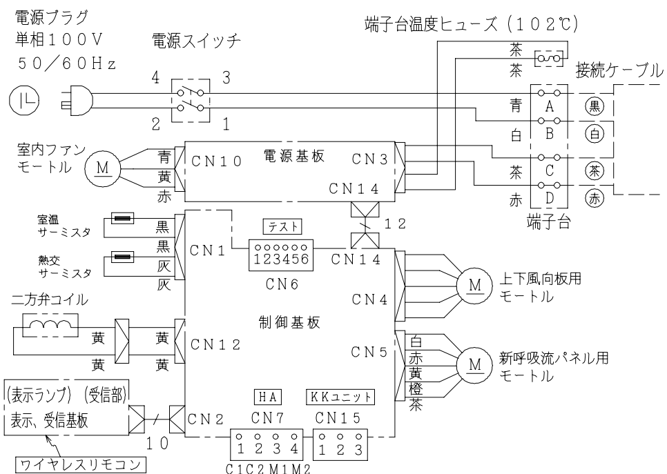
配線図 RAS-289HX
