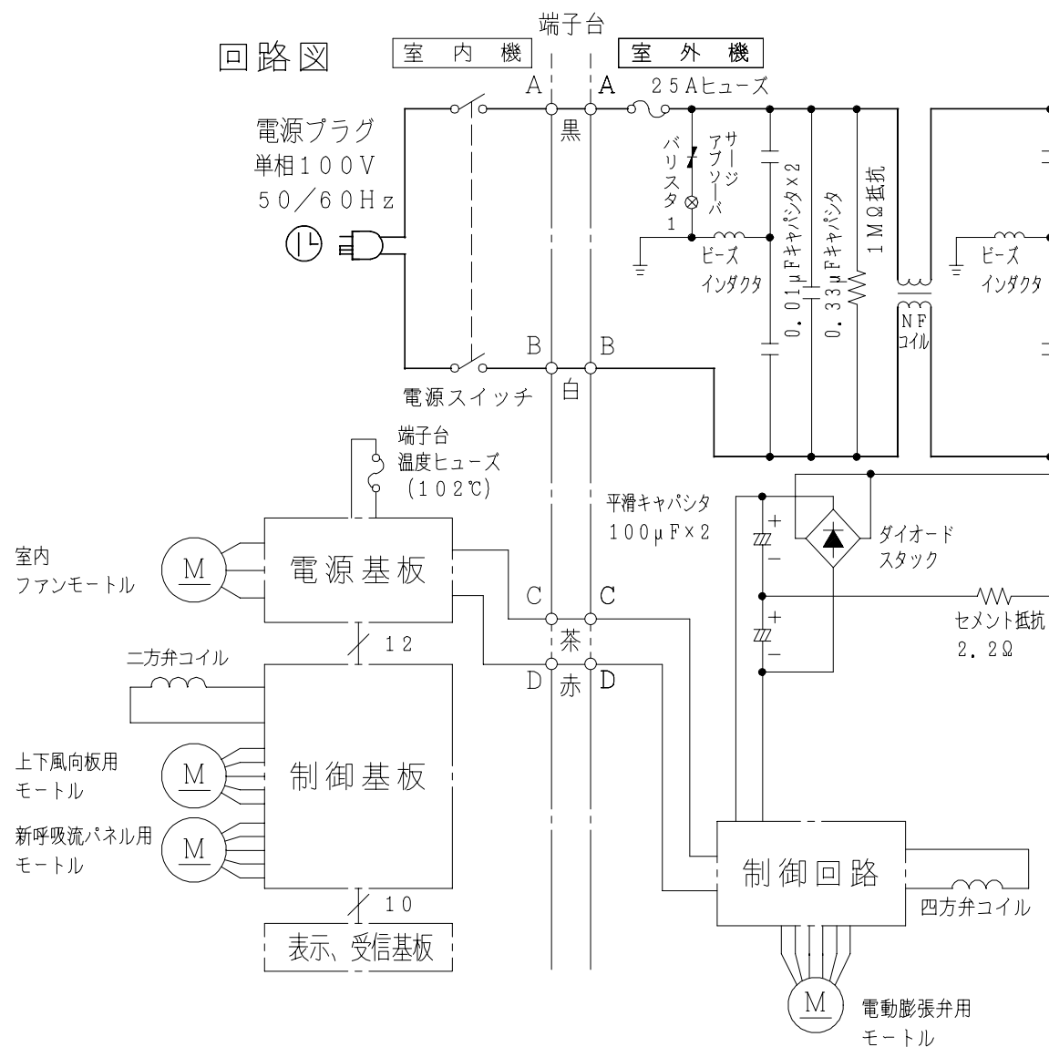
配線図 RAS-289HX
