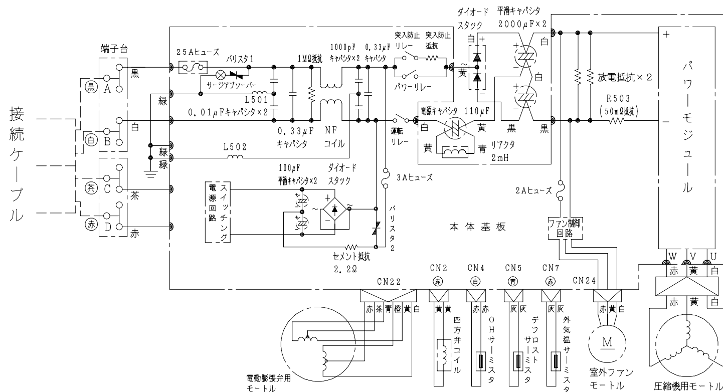
配線図 RAC-289HX
