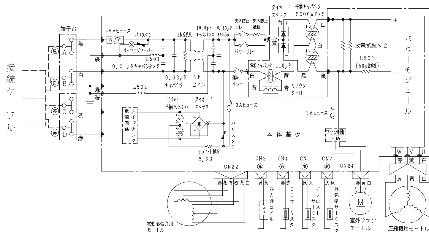
配線図 RAC-289GX
