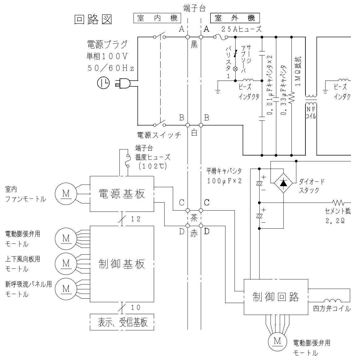
配線図 RAS-289GX
