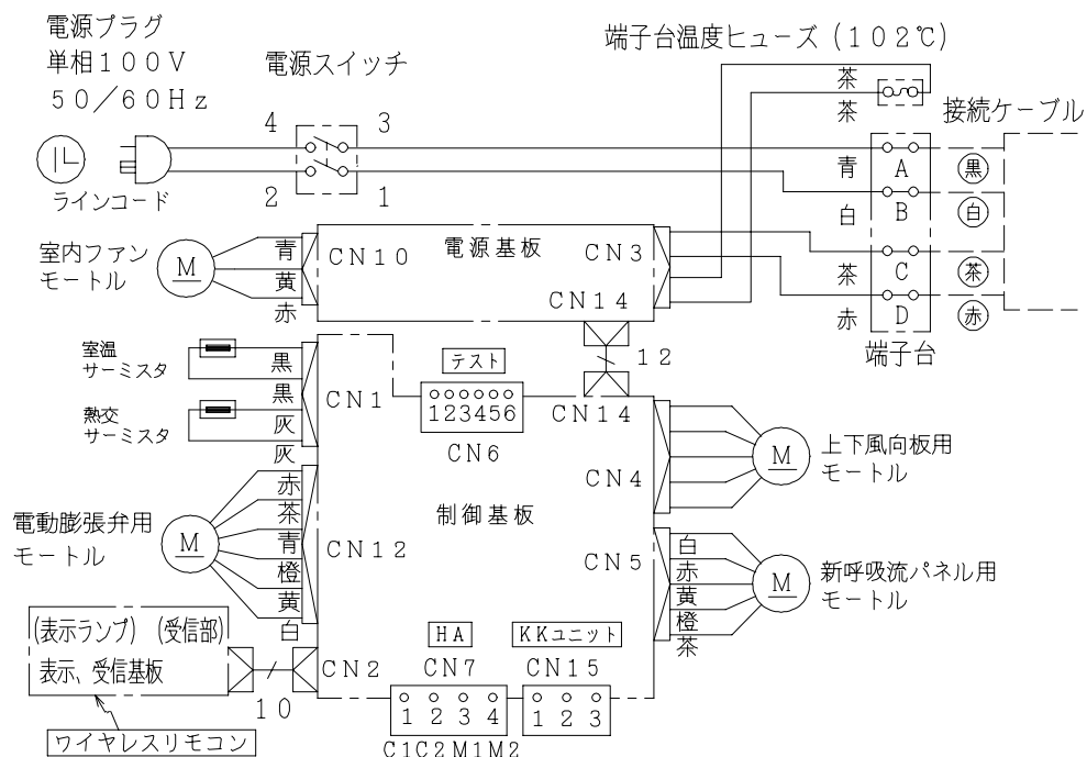
配線図 RAS-289GX
