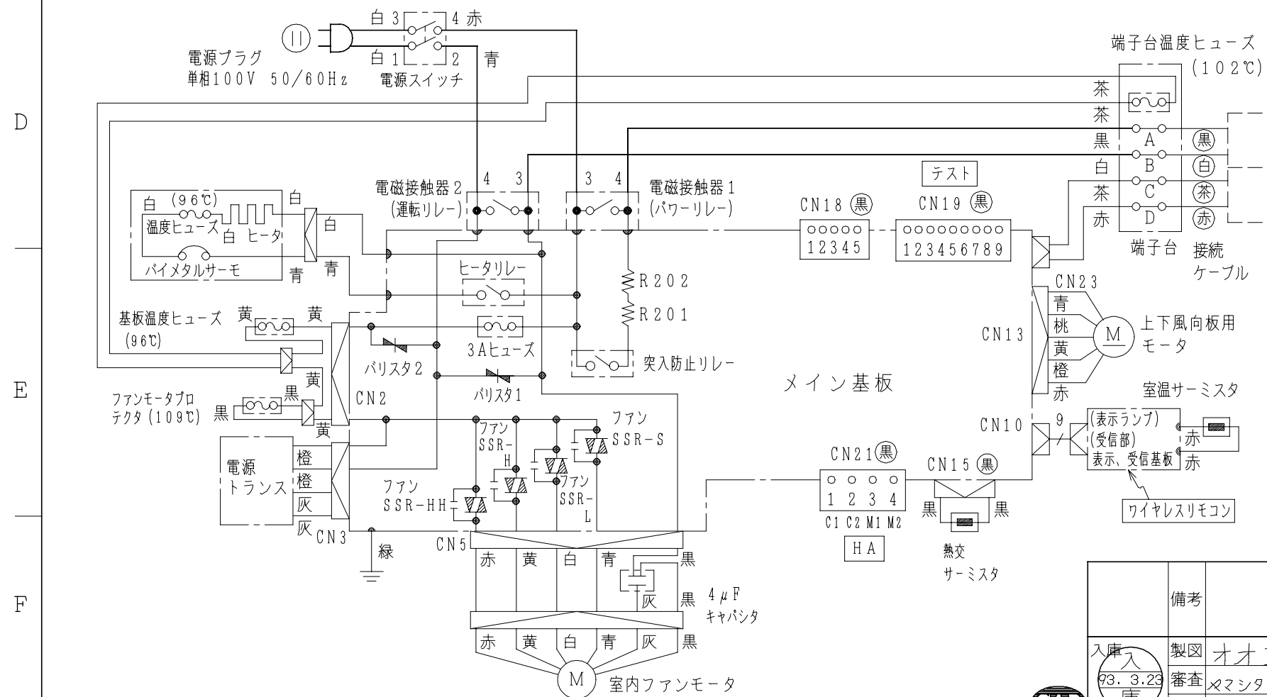
配線図 RAS-289DE
