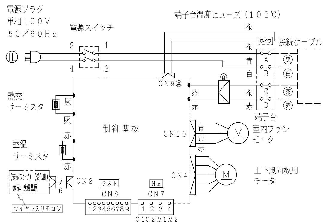
配線図 RAS-288GX
