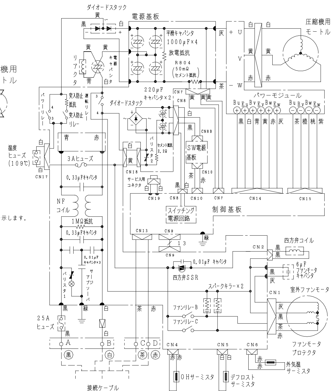
配線図 RAC-28GX
