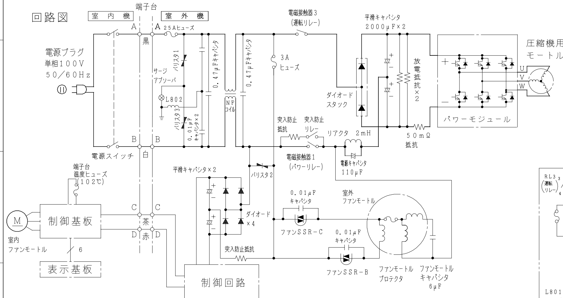
配線図 RAS-287GE
