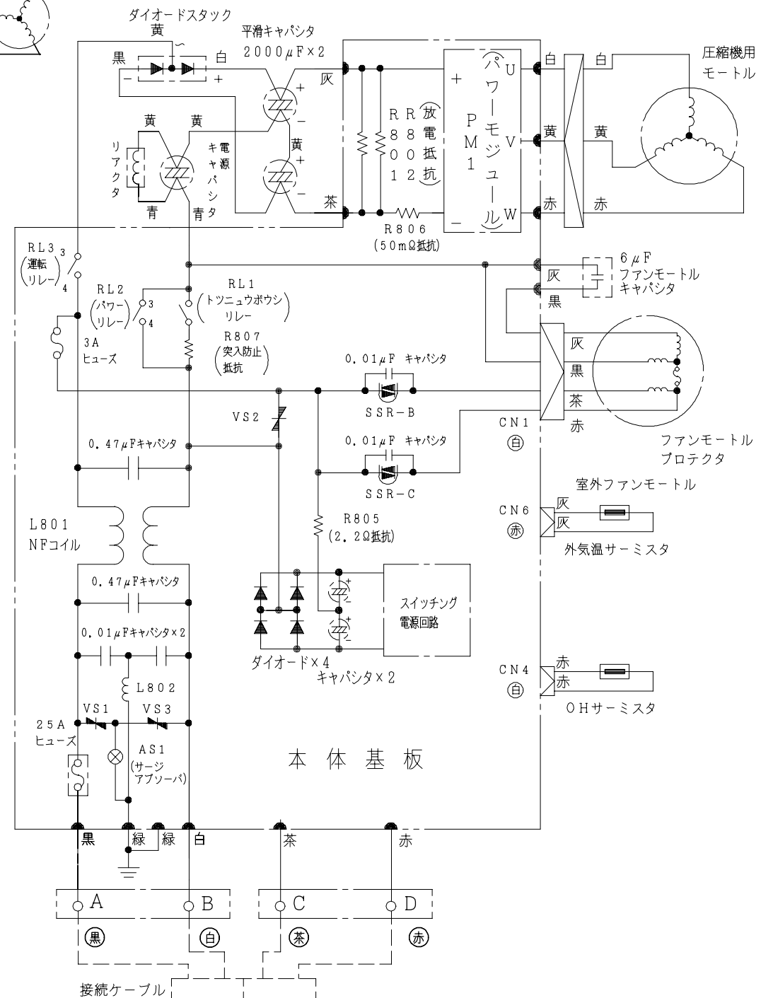
配線図 RAC-287GE
