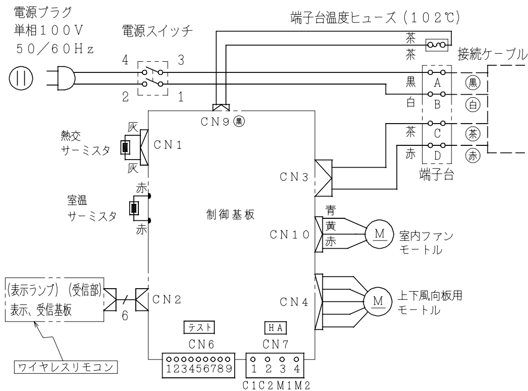
配線図 RAS-287GE
