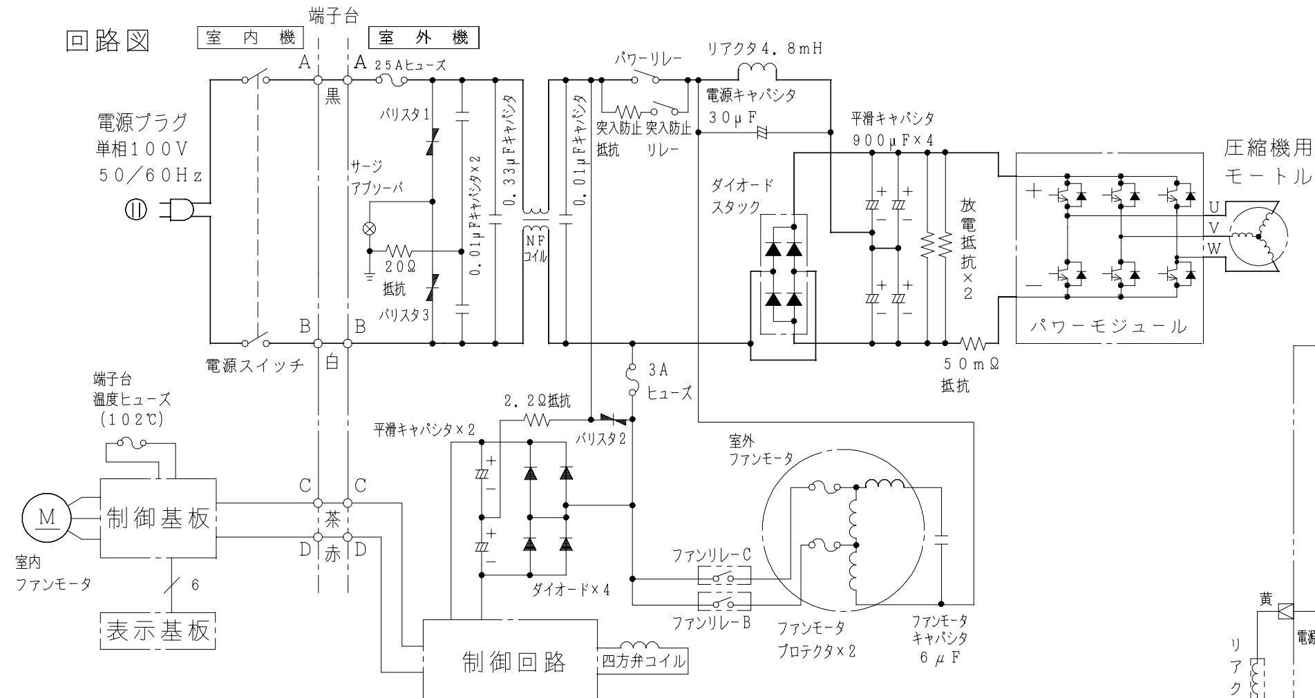
配線図 RAS-25SJX
