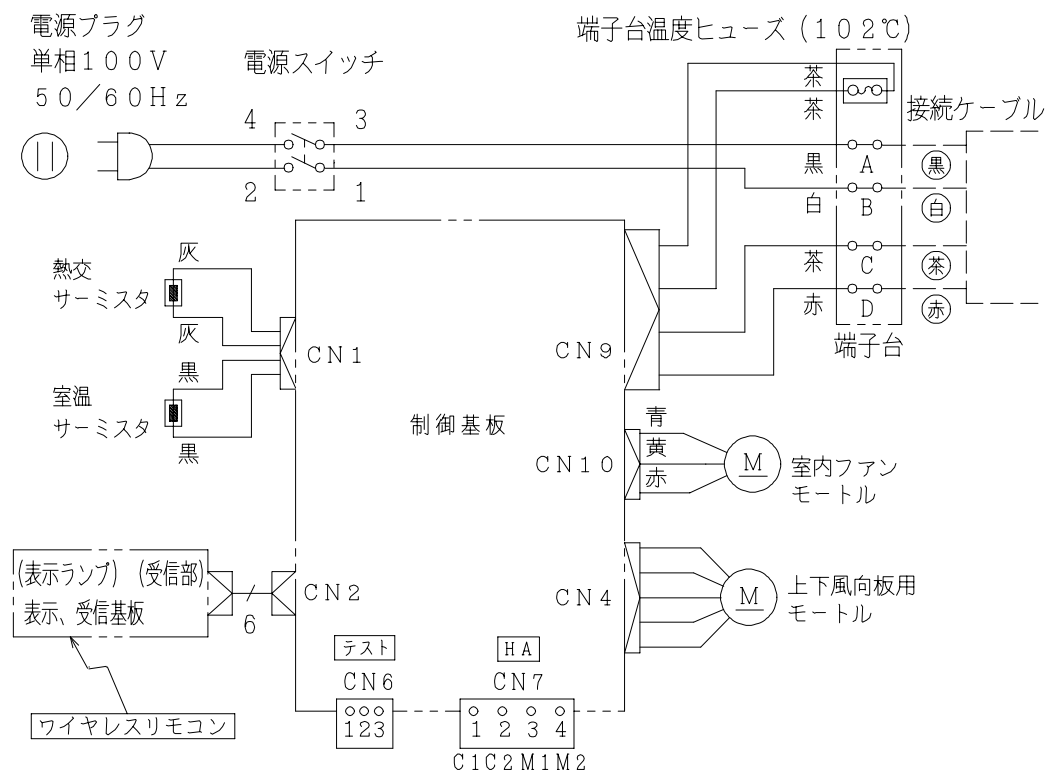
配線図 RAS-25SJX
