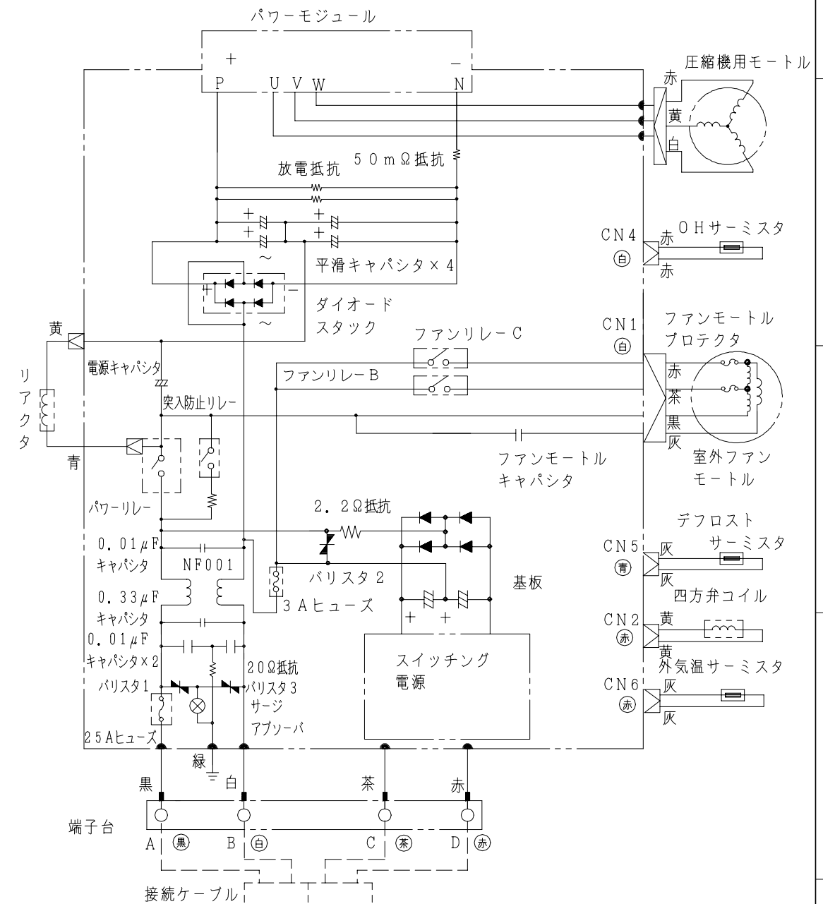
配線図 RAC-25SJX
