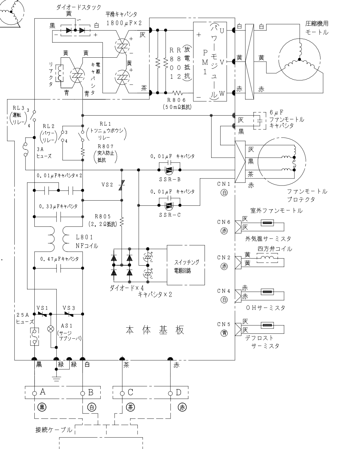
配線図 RAC-25HSGX
