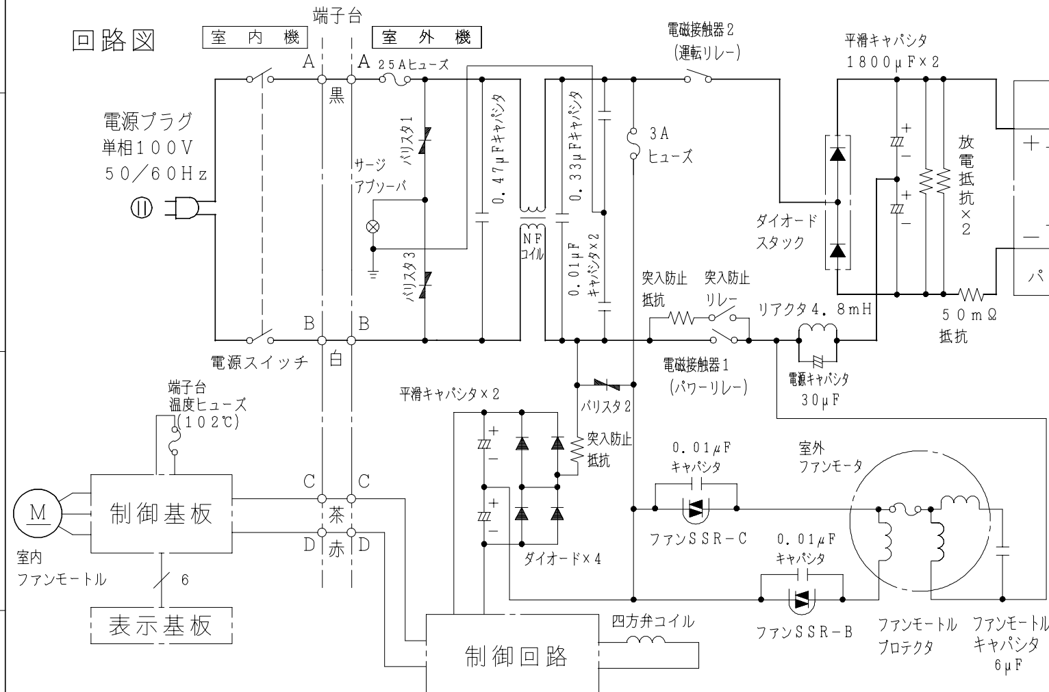
配線図 RAS-25SGX
