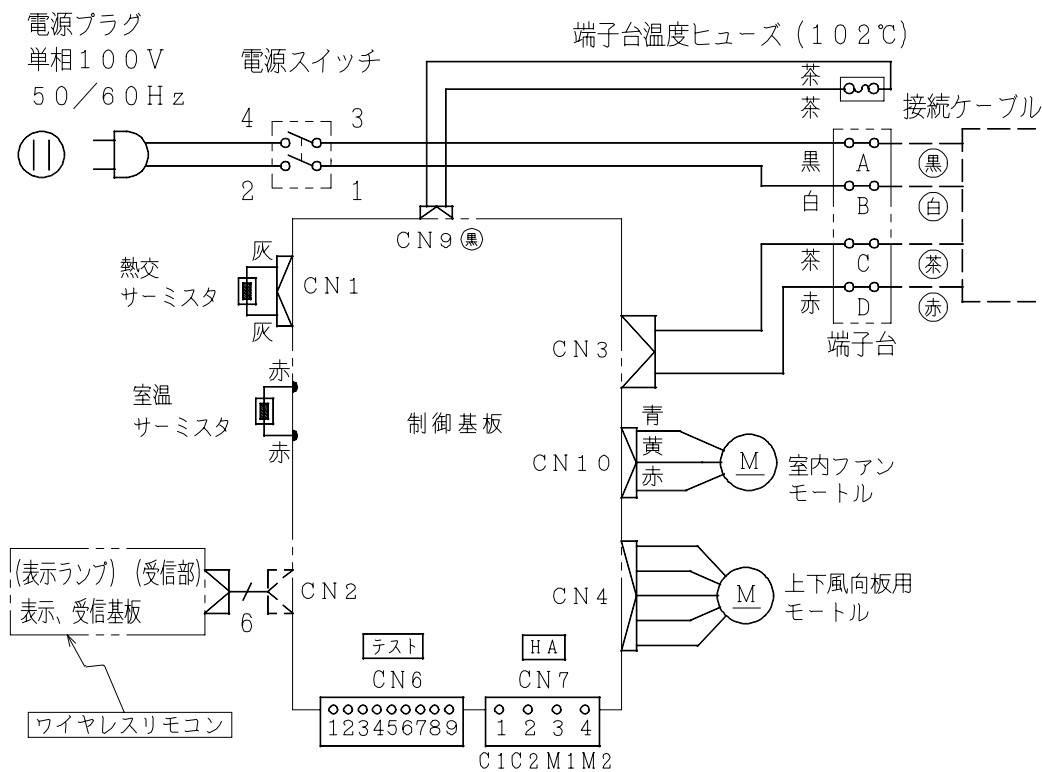
配線図 RAS-25SGX
