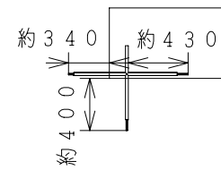
背面から見る (配管引出寸法)
