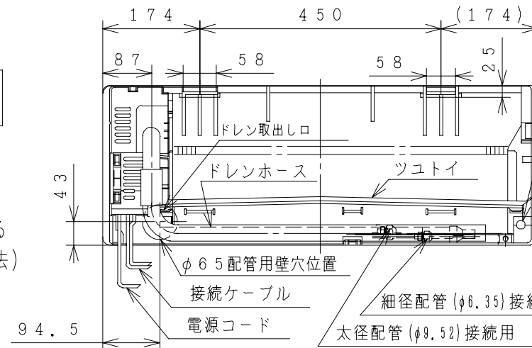
背面図
