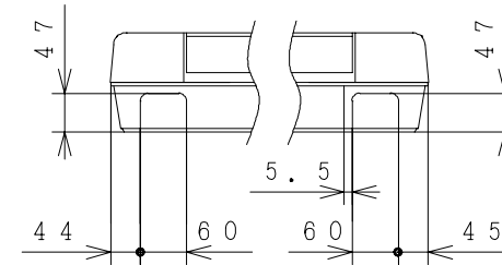
Pから見る（下引配管位置）
