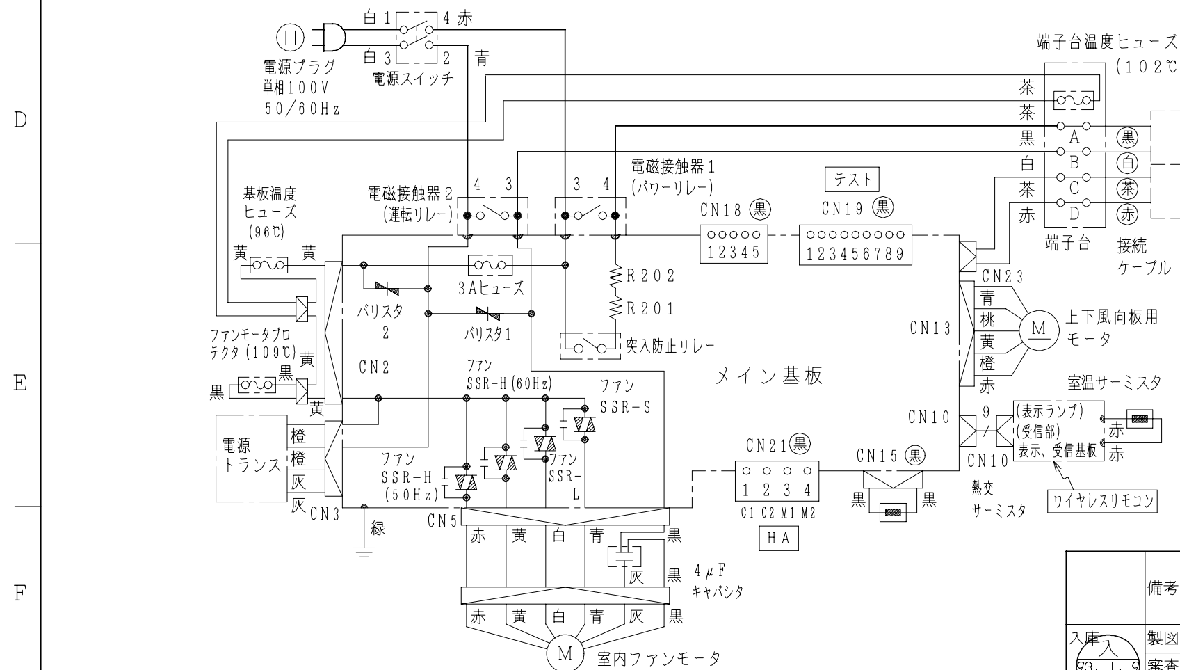
配線図 RAS-25DXC
