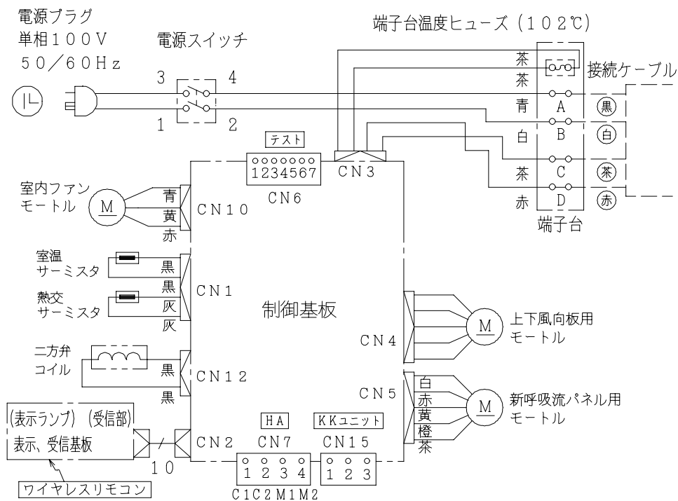
配線図 RAS-259HX
