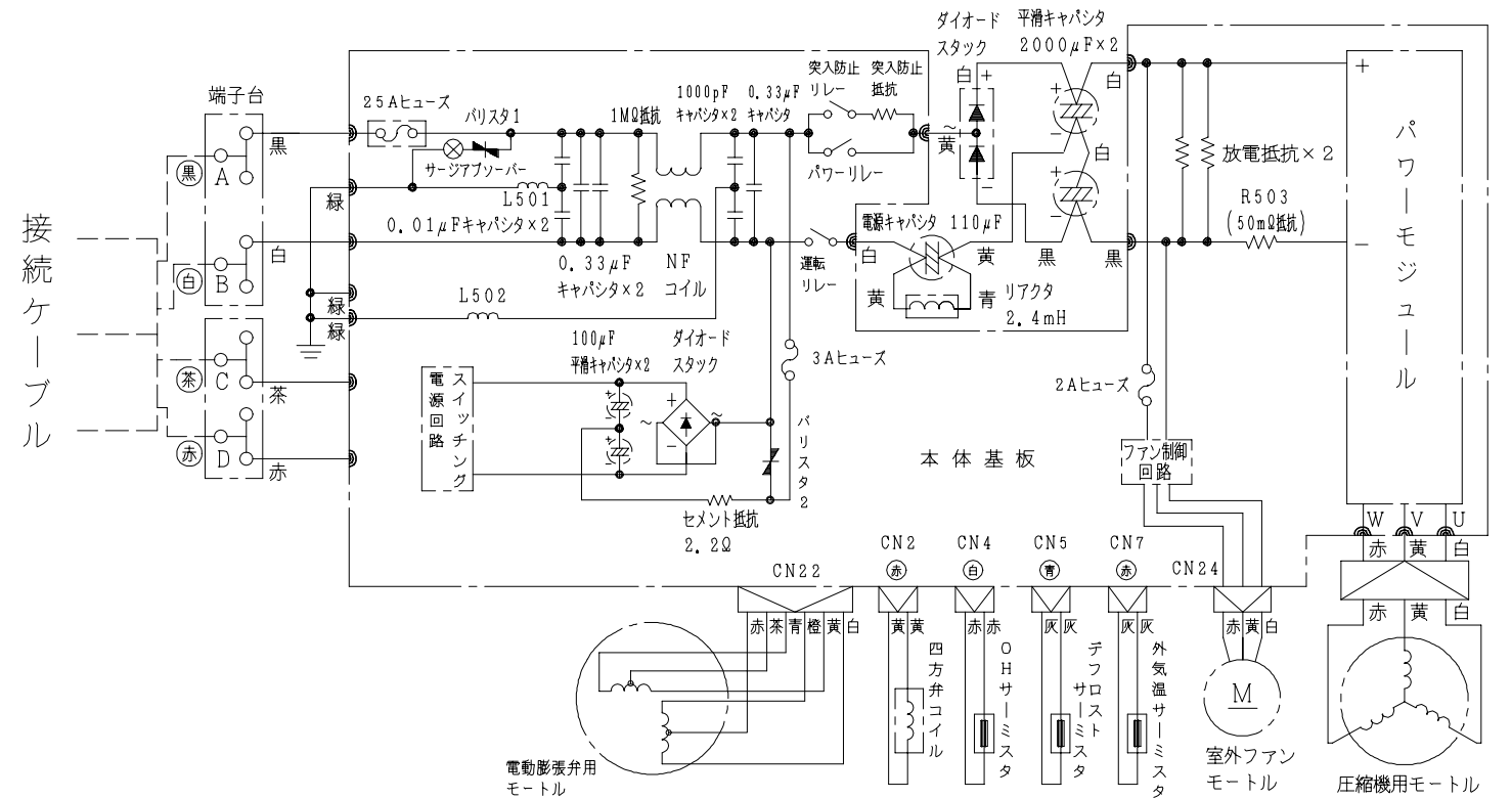
配線図 RAC-259HX
