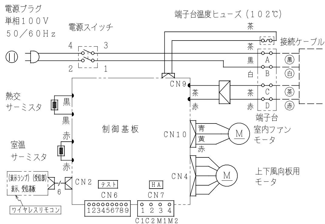
配線図 RAS-258EX
