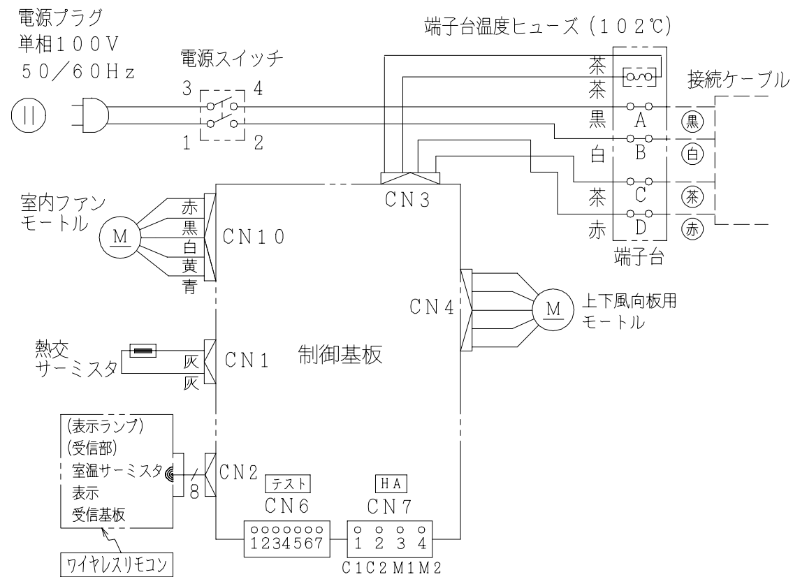
配線図 RAS-22RX
