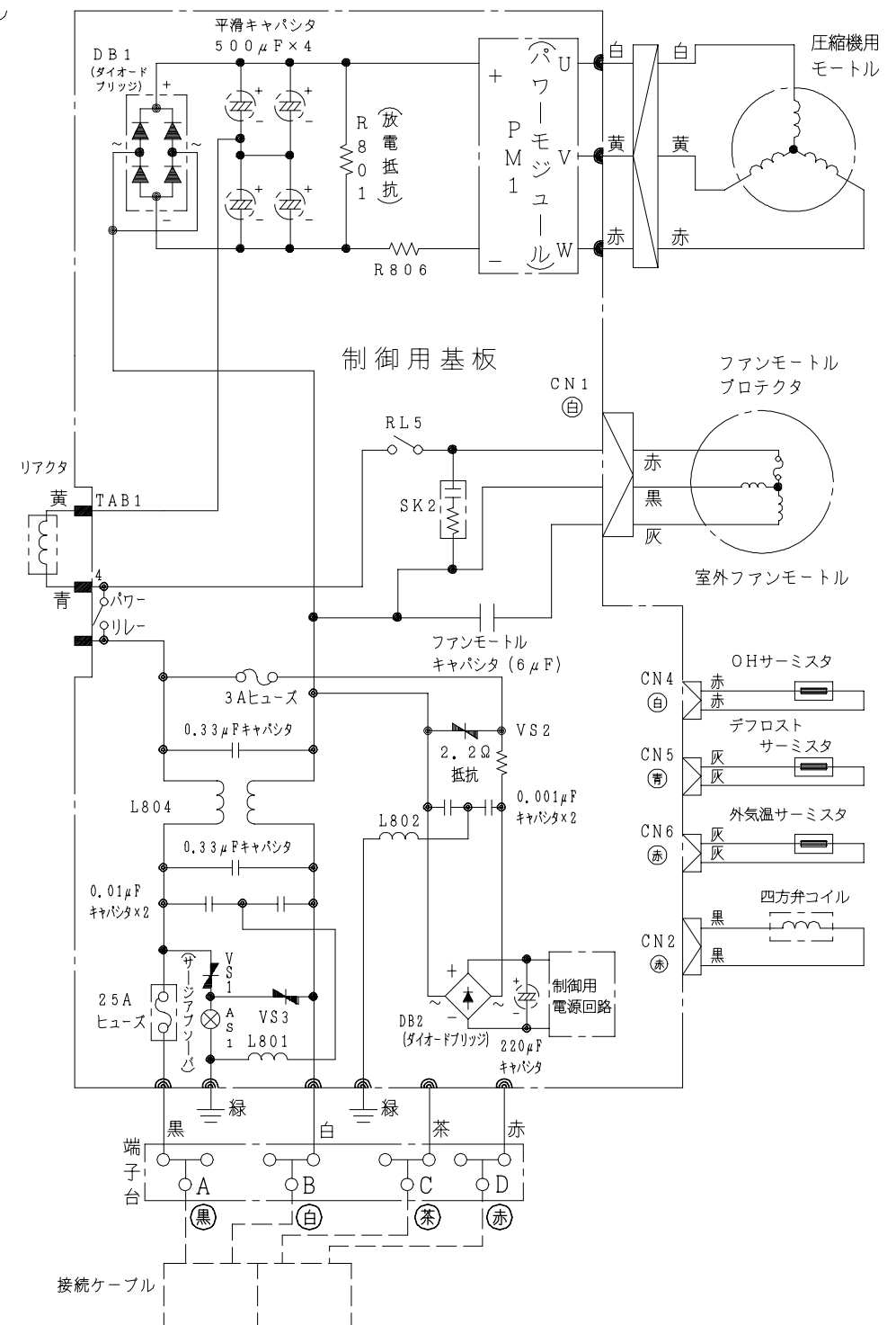
配線図 RAC-22RX
