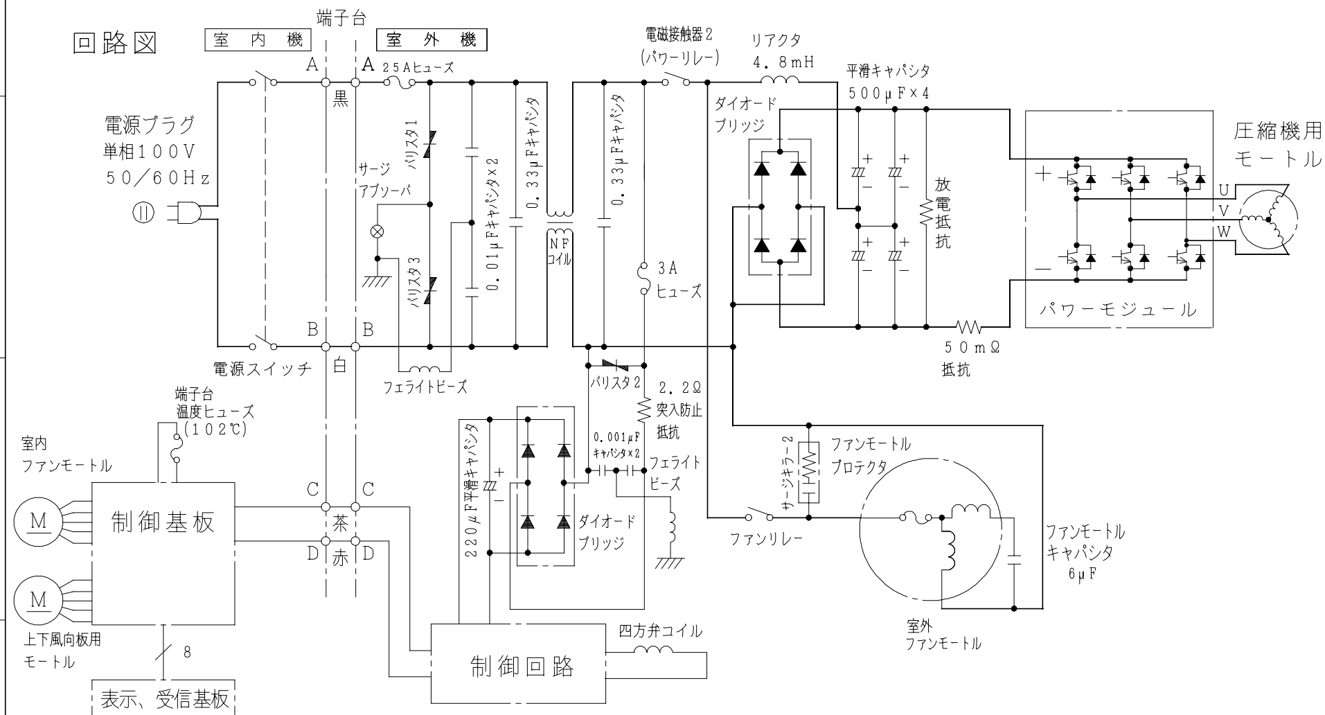
配線図 RAS-22RX
