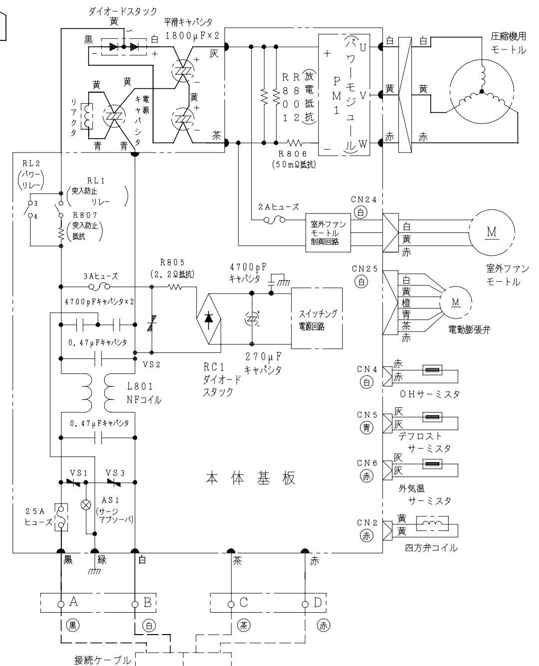
配線図 RAC-22HJX
