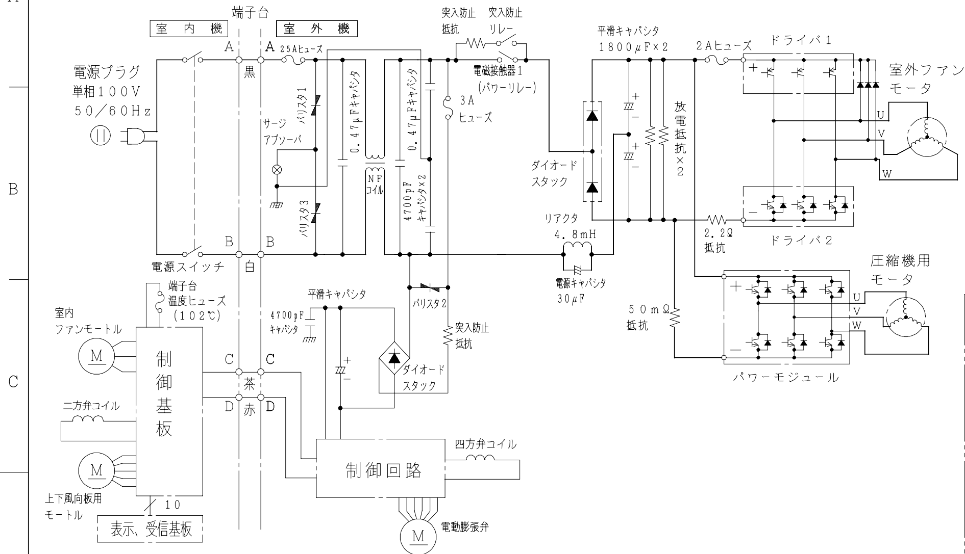
回路図
