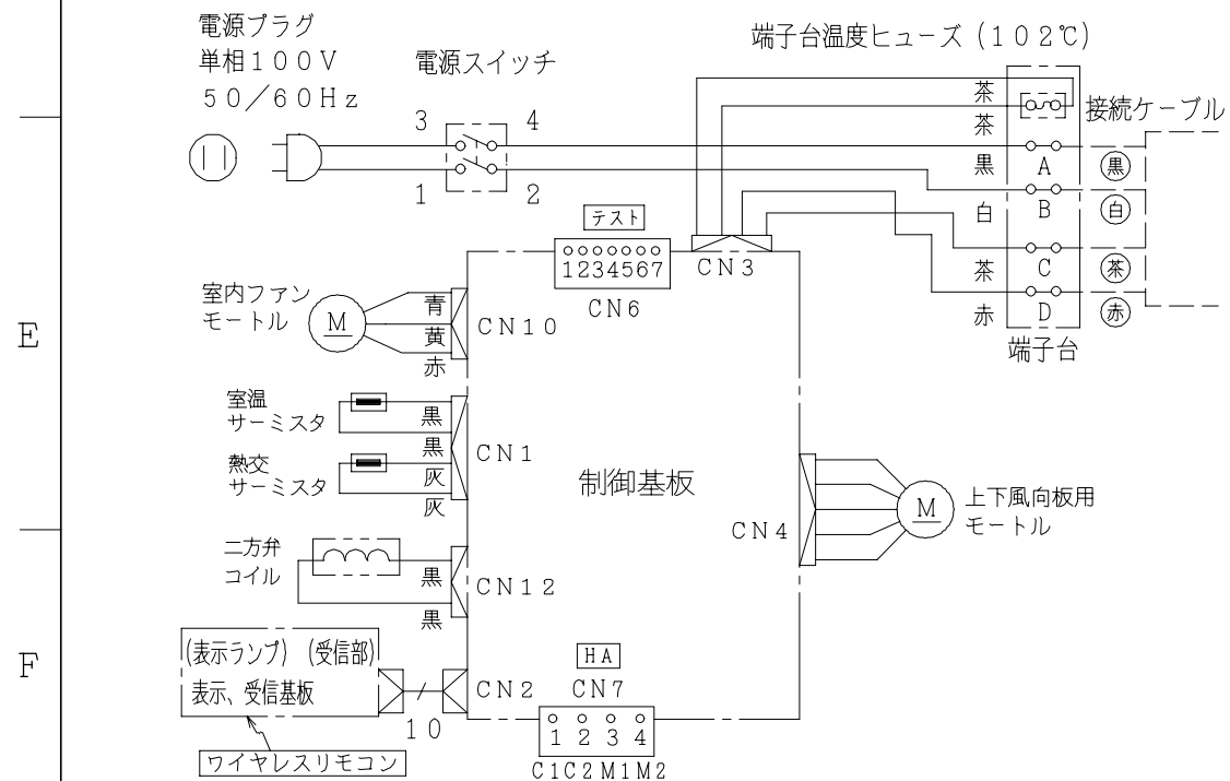
配線図 RAS-22HJX
