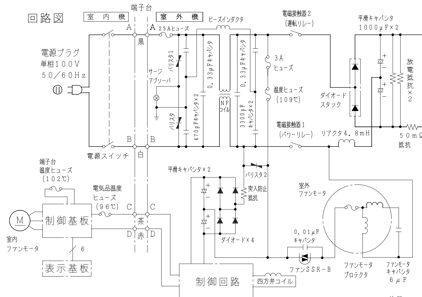
配線図 RAS-22FXR
