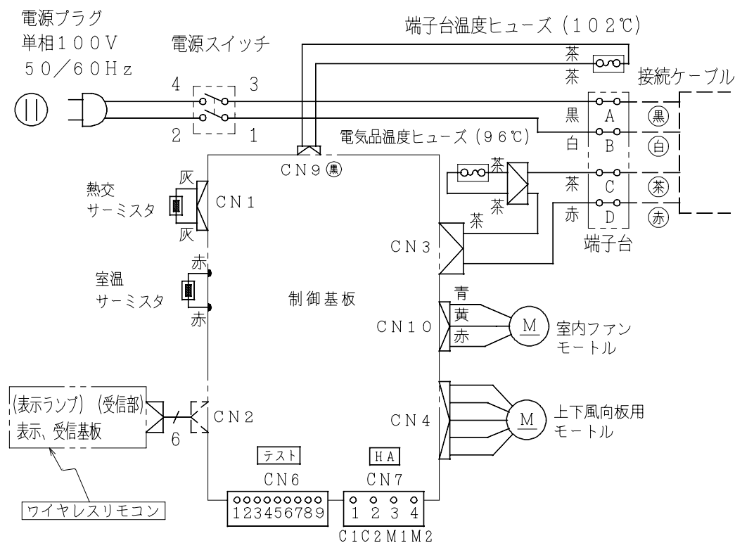
配線図 RAS-22FXR
