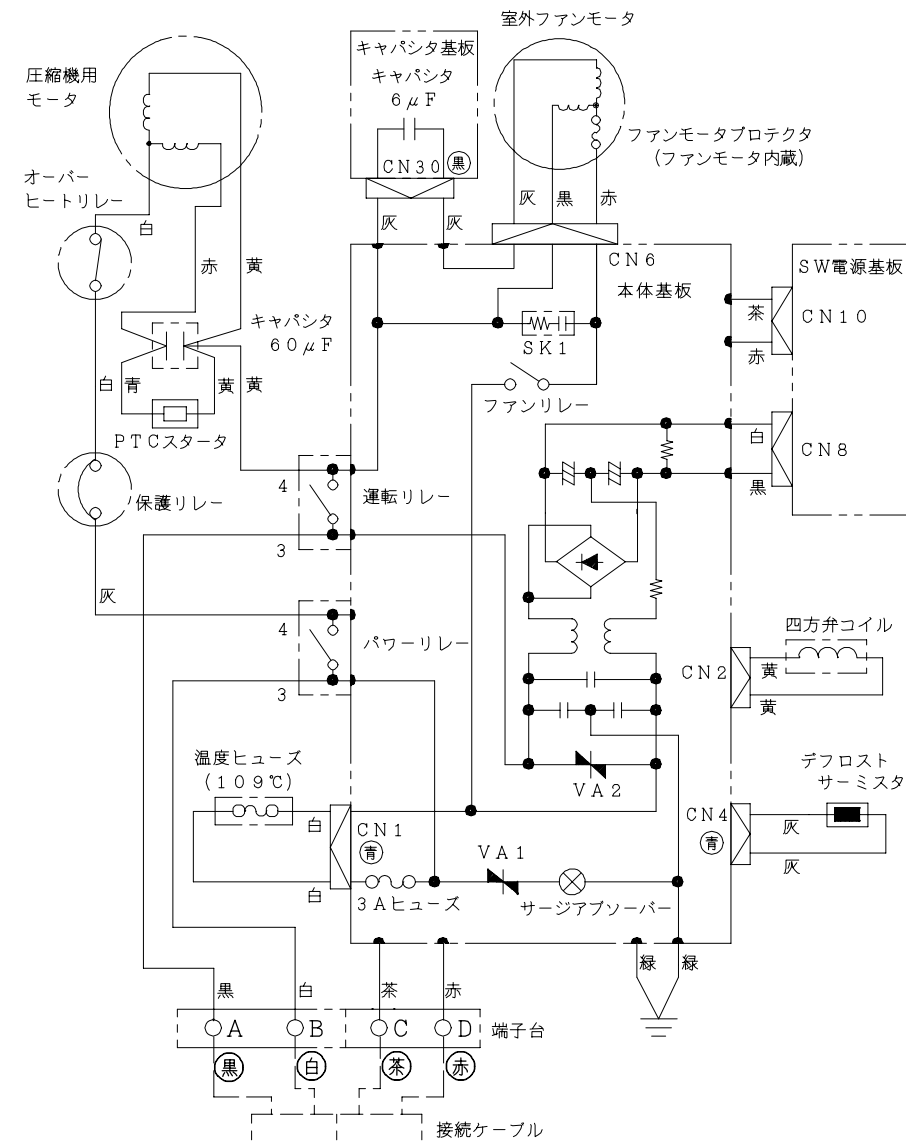
配線図
