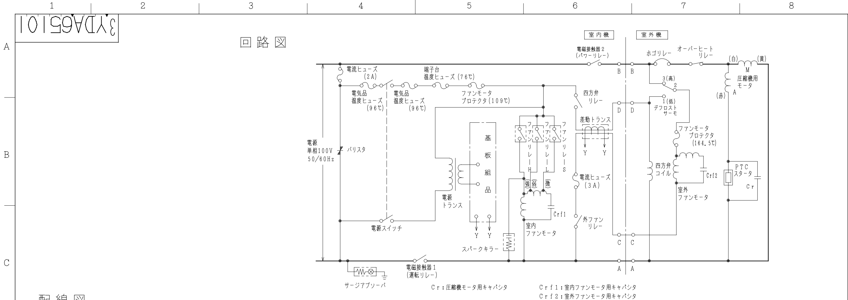
配線図
