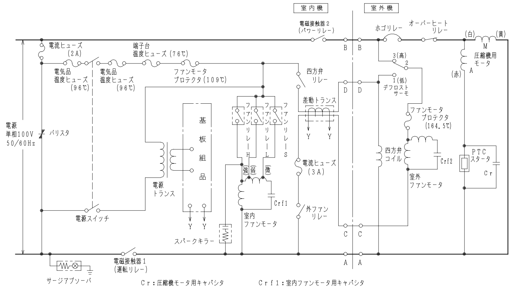
回路図
