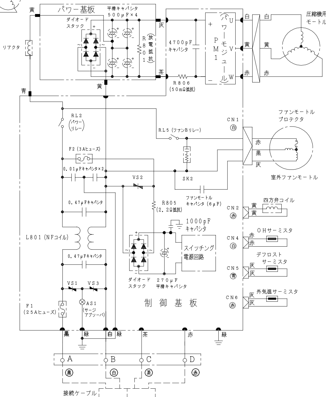
配線図 RAC-228LX
