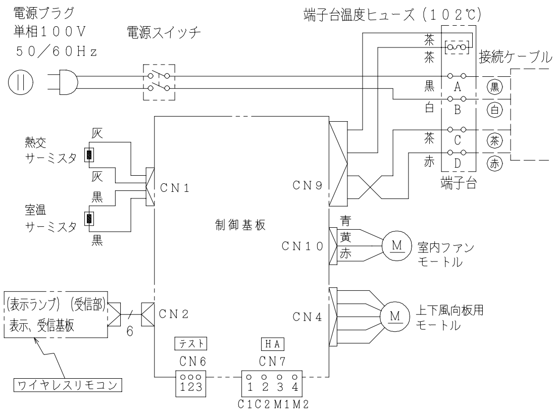
配線図 RAS-228LX
