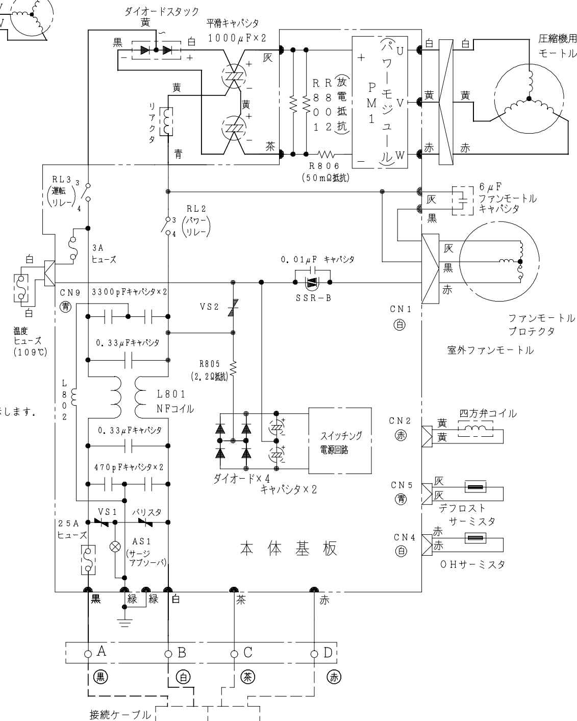
配線図 RAC-22FX
