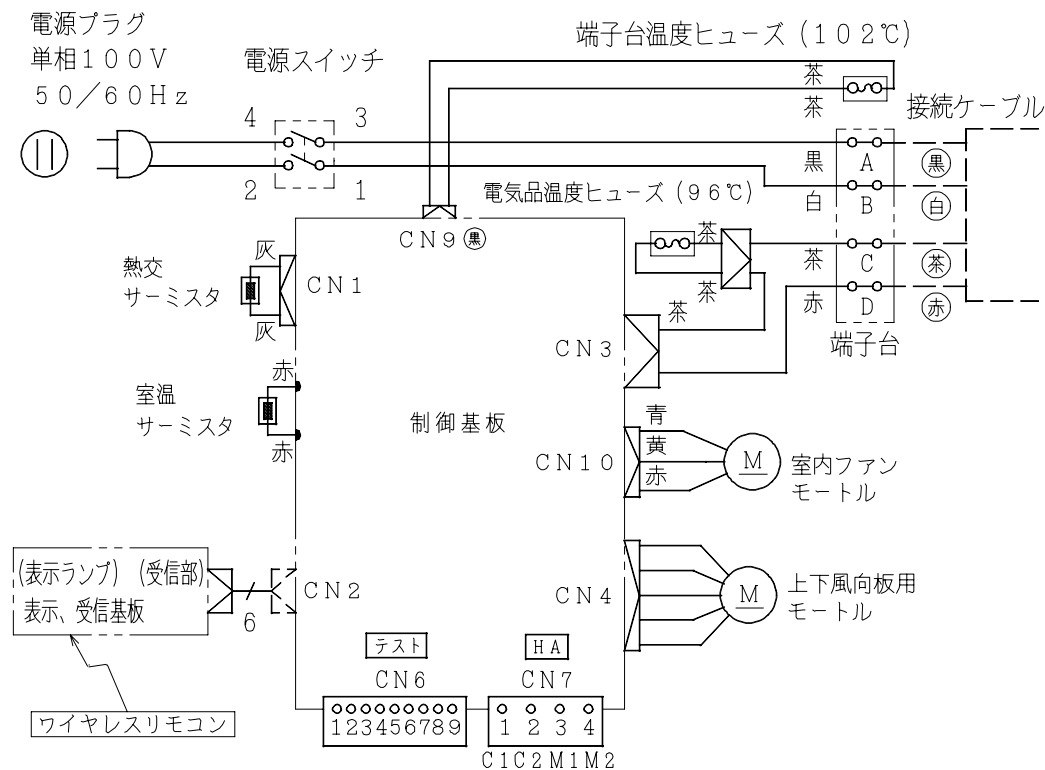
配線図 RAS-228FX
