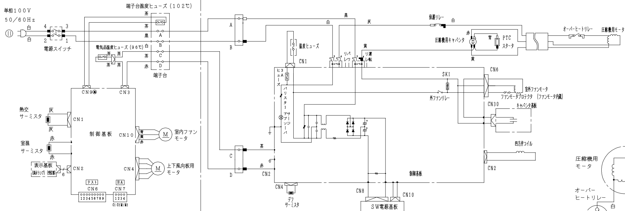
回路図
