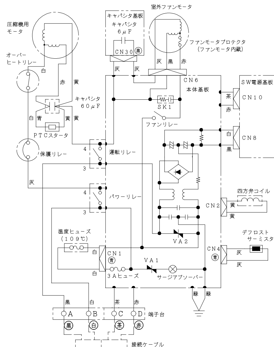
配線図
