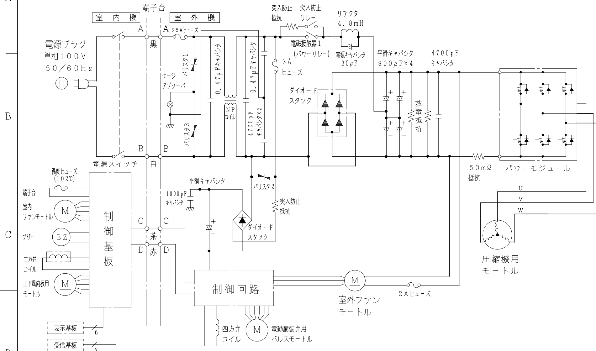
配線図 RAS-20LEM
