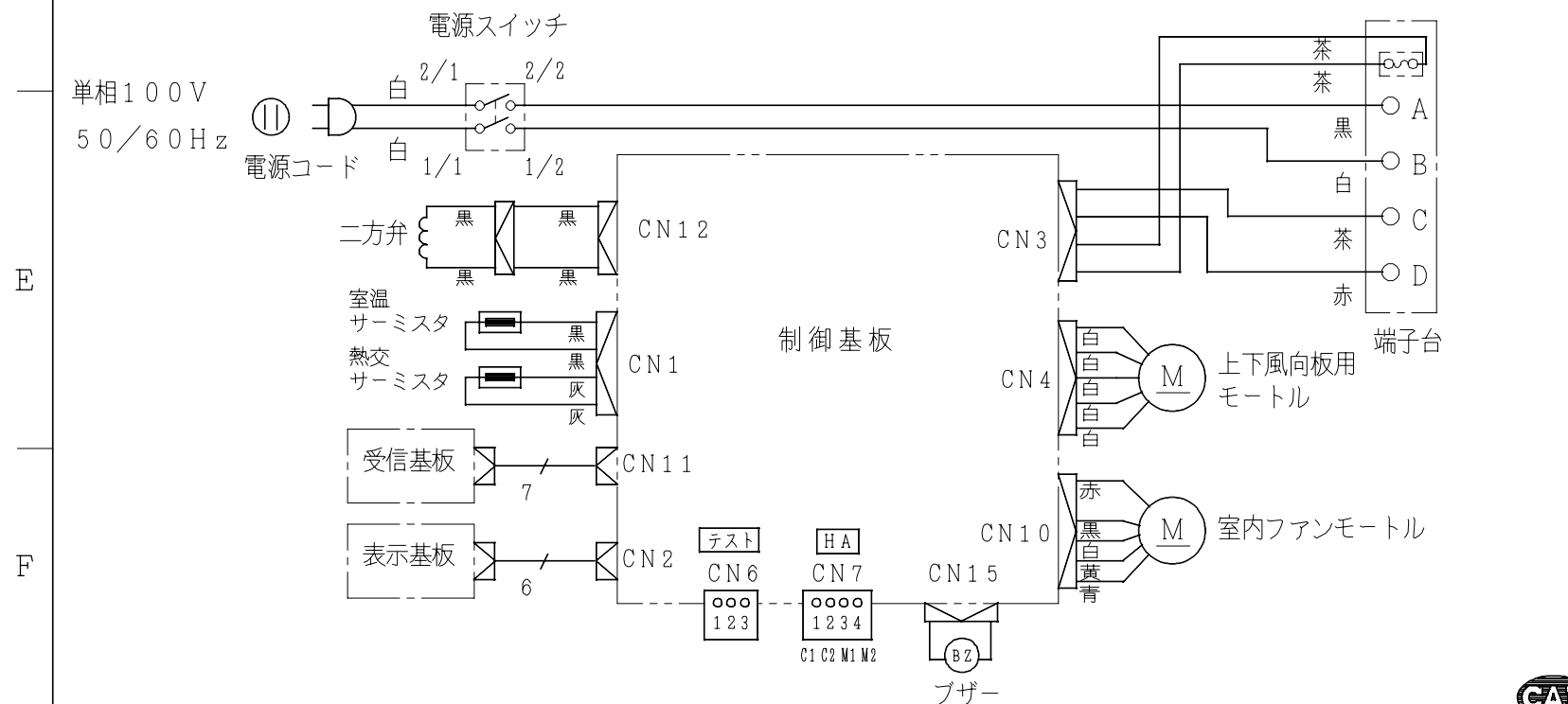
配線図 RAS-20LEM
