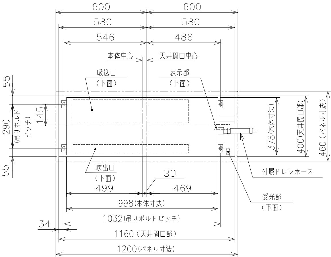
日立ルームエアコン ー方向天井カセットPAシリーズ 室内ユニット 寸法図
