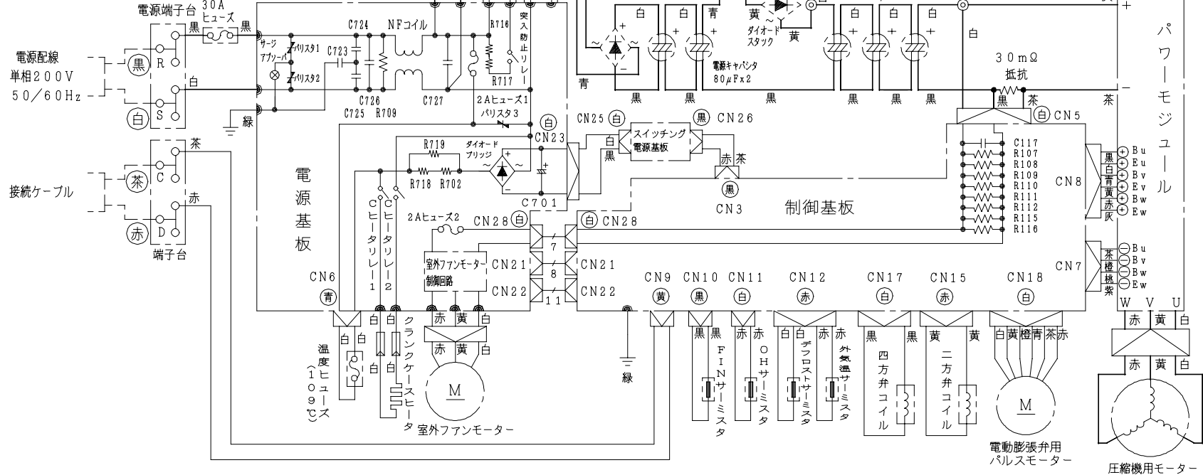
室外機配線図
