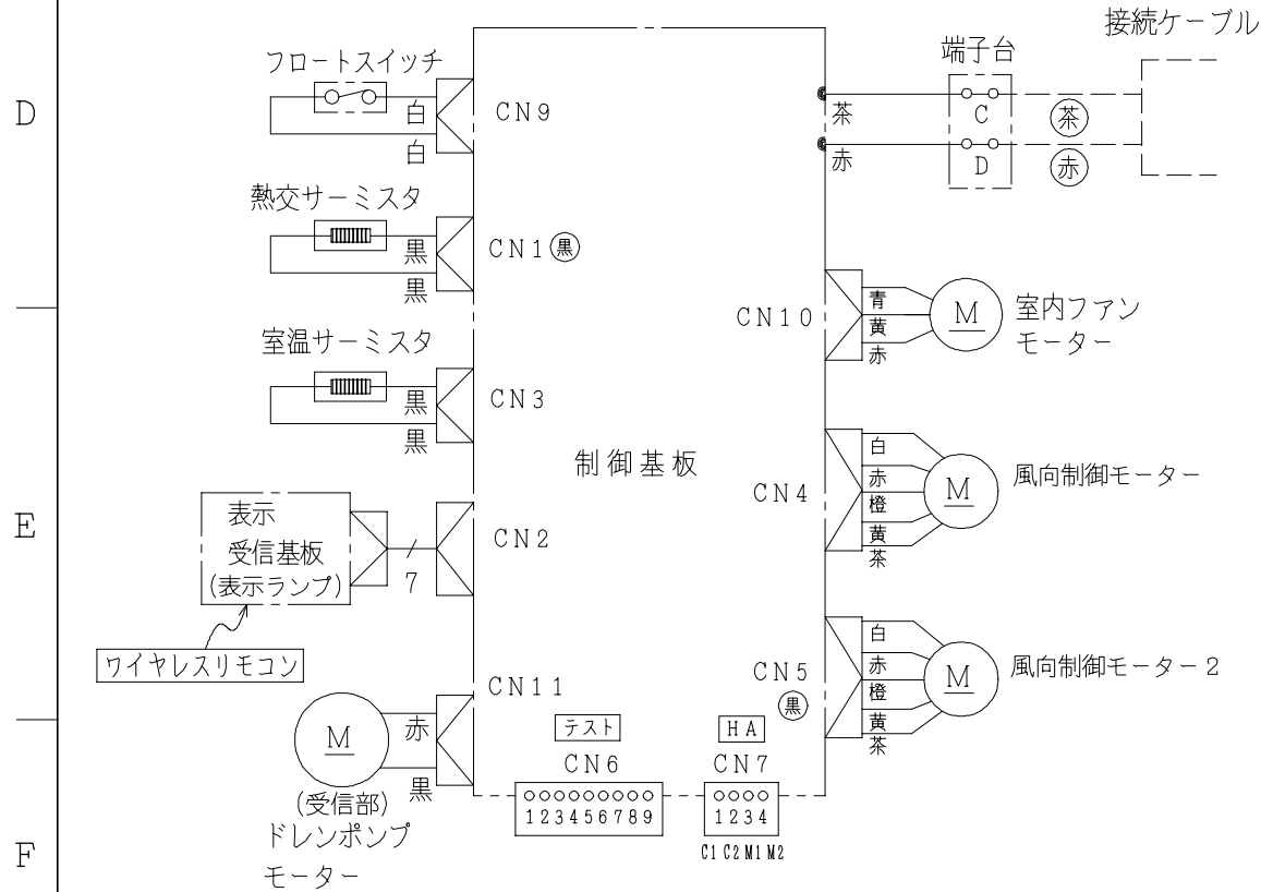
室内機配線図
