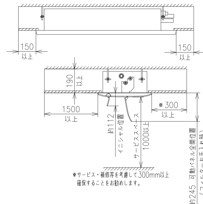
据付必要寸法図
