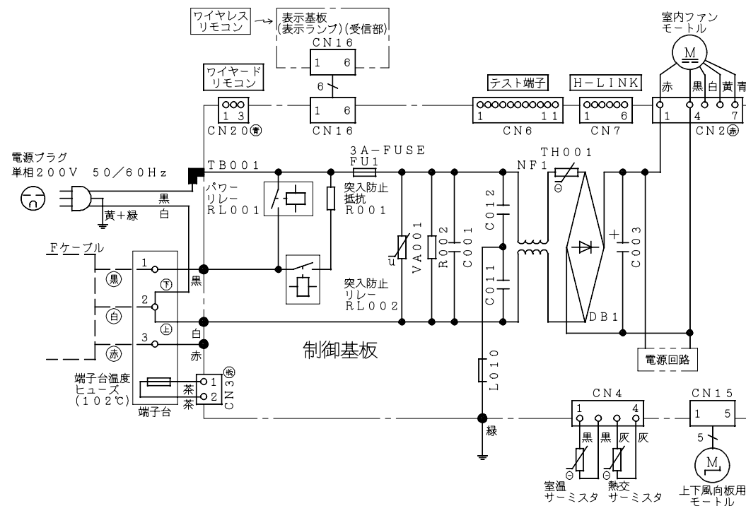
配線図 RAS-AJ28D2
