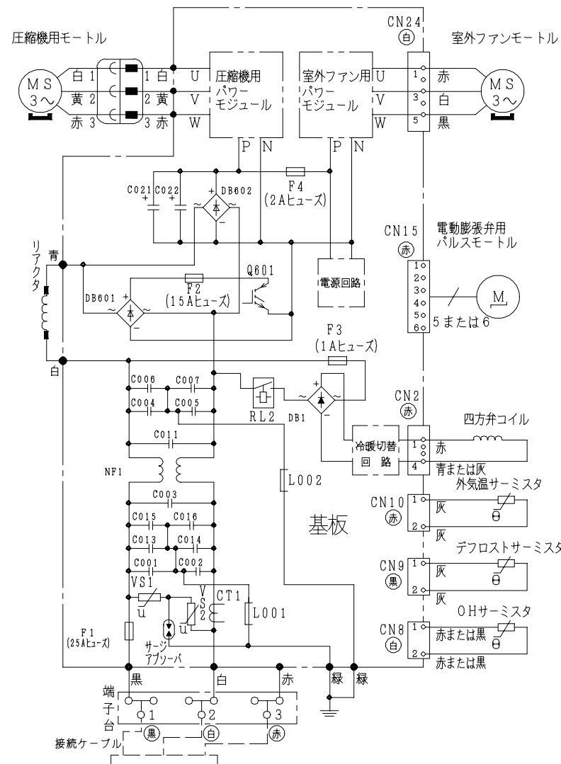
配線図 RAC-AJ28D2
