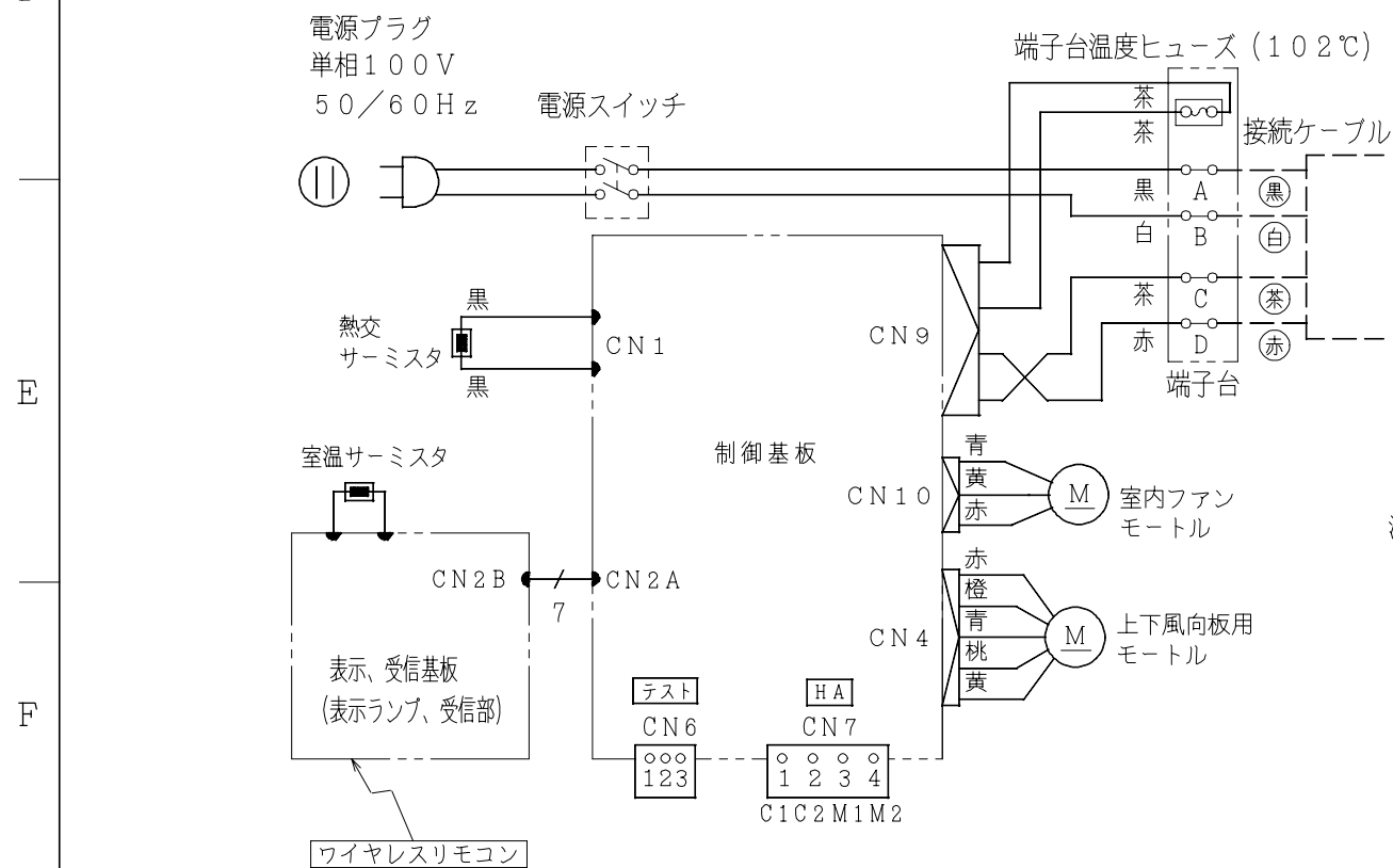
配線図 RAS-22MX
