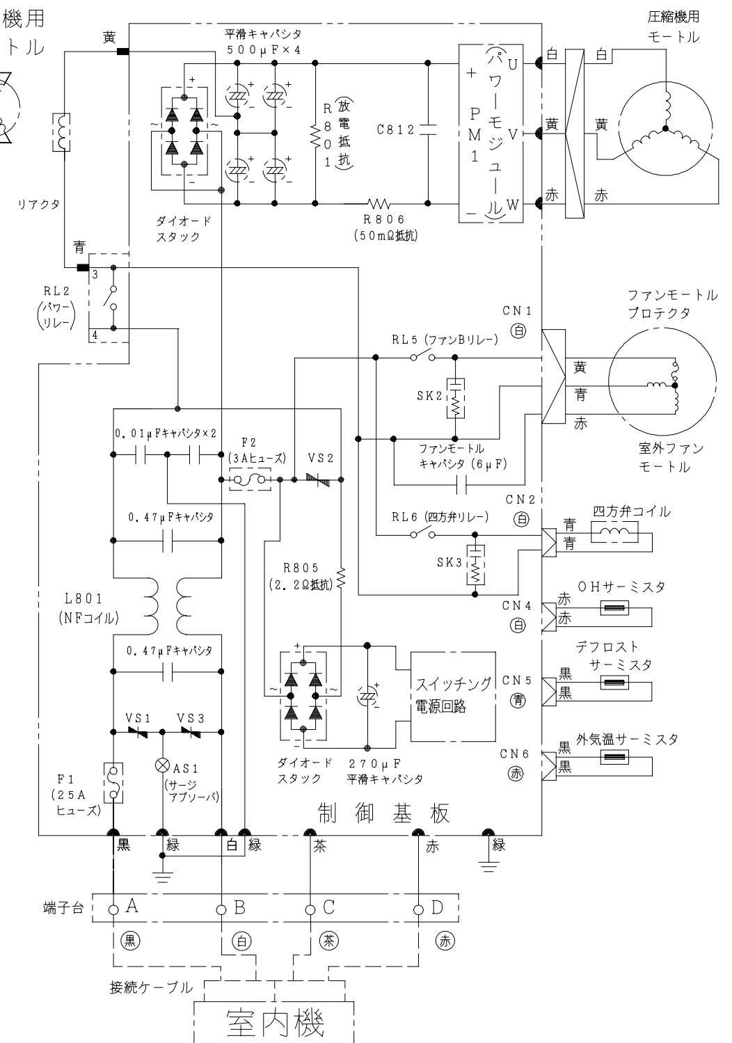
配線図 RAC-22MX
