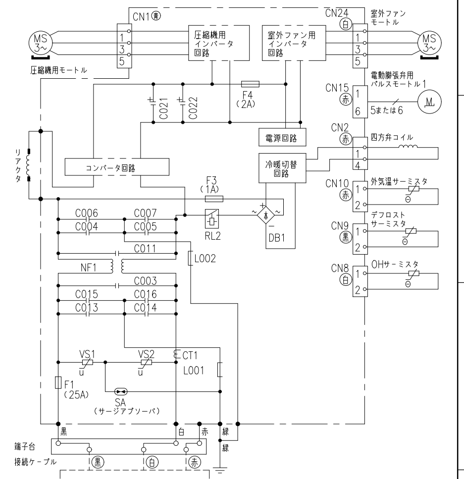
配線図 RAC-MJ56K2EE
