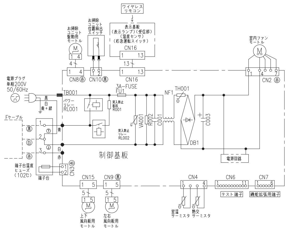
配線図 RAS-MJ56K2EE
