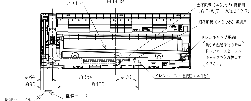
背面図
