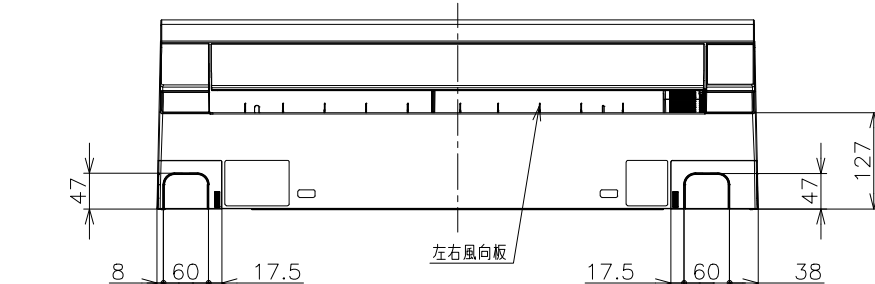
背面図
