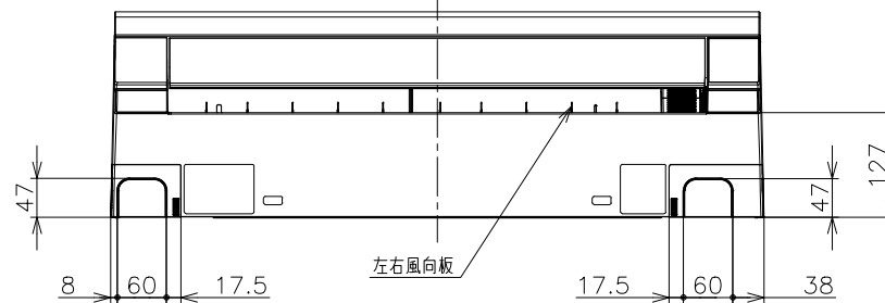
背面図
